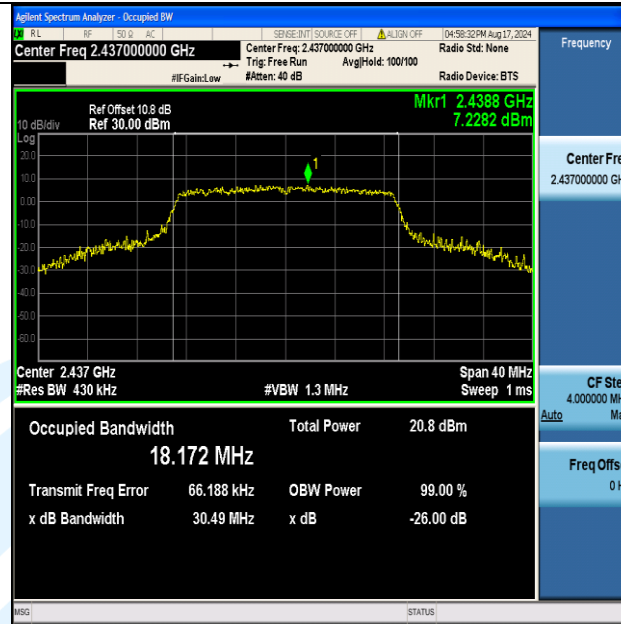
11N20MIMO-Ant2-2437
