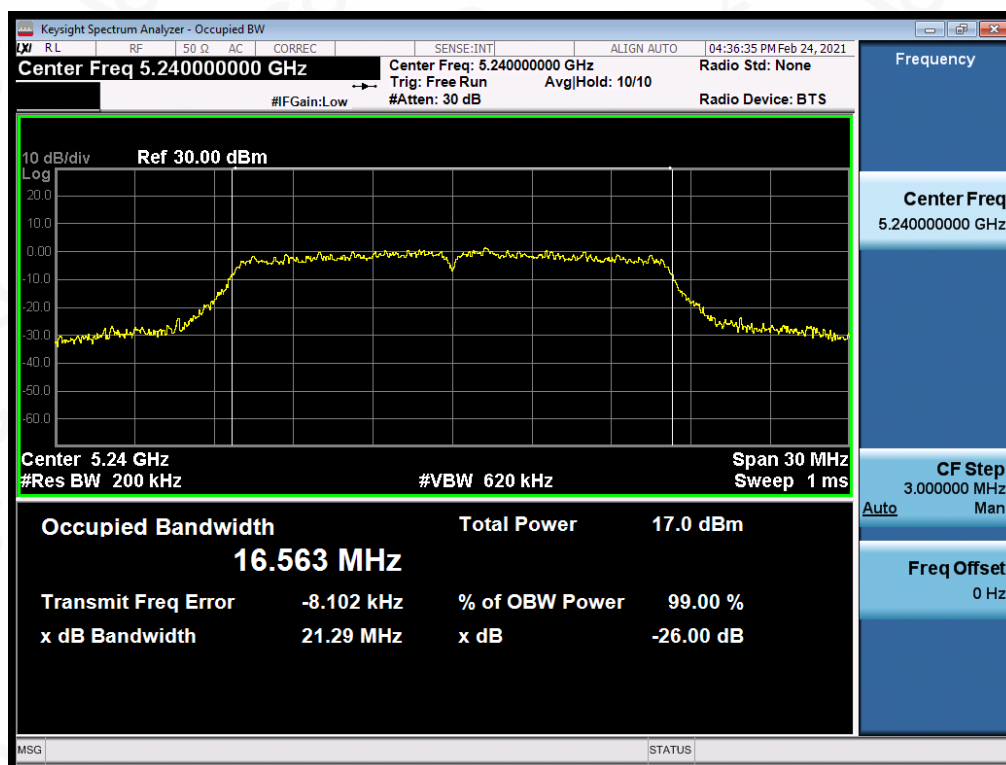
Test_Graph_802.11a_ANT1_5240_6Mbps_OBW
