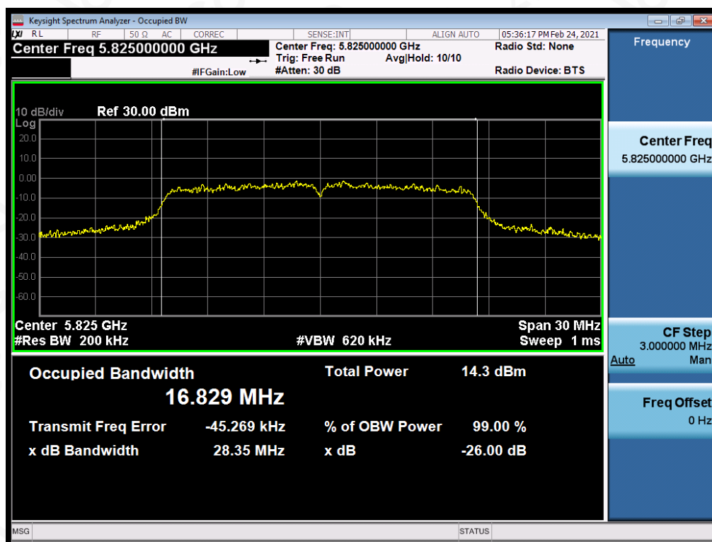
Test_Graph_802.11a_ANT1_5825_6Mbps_OBW
