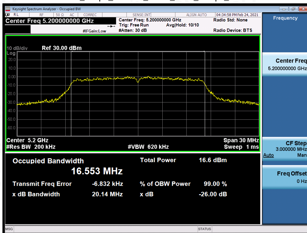
Test_Graph_802.11a_ANT1_5200_6Mbps_OBW
