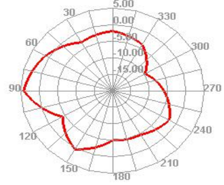
5500.000MHz H
