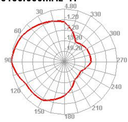
5150.000MHz H
