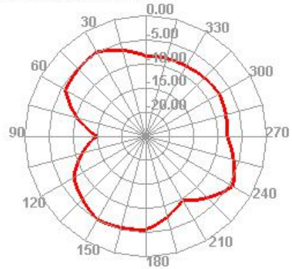
2410.000MHz H
