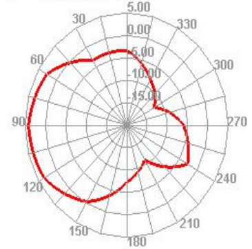
5500.000MHz E2
