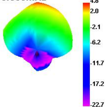
5150.000MHz
