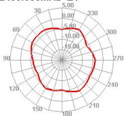
2480.000MHz E1
