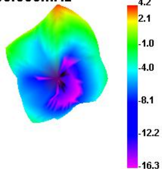
5500.000MHz
