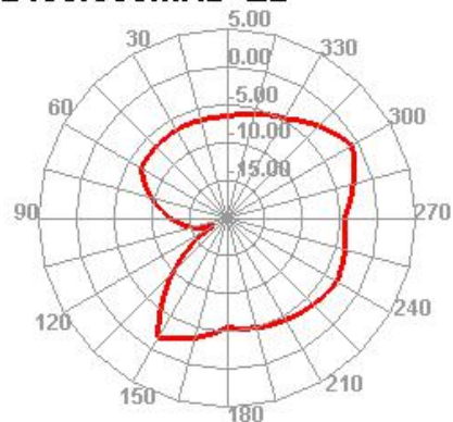
2480.000MHz E2
