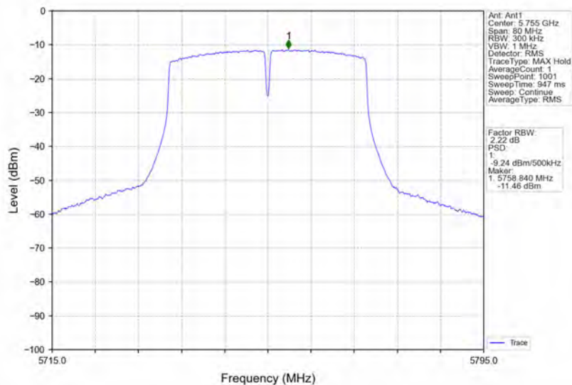
802.11n(HT40)_LCH_5755MHz_Ant1_NTNV
