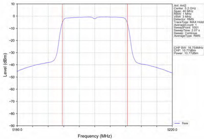
802.11a_MCH_5200MHz_Ant2_NTNV
