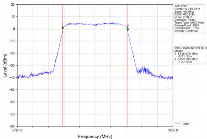
802.11a_LCH_5745MHz_Ant2_NTNV
