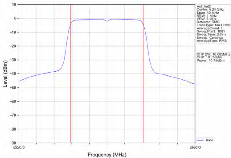
802.11a_HCH_5240MHz_Ant2_NTNV
