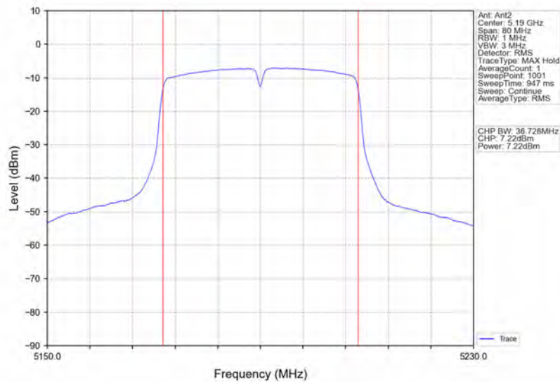
802.11n(HT40)_LCH_5190MHz_Ant2_NTNV
