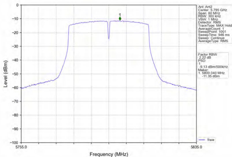
802.11n(HT40)_HCH_5795MHz_Ant2_NTNV
