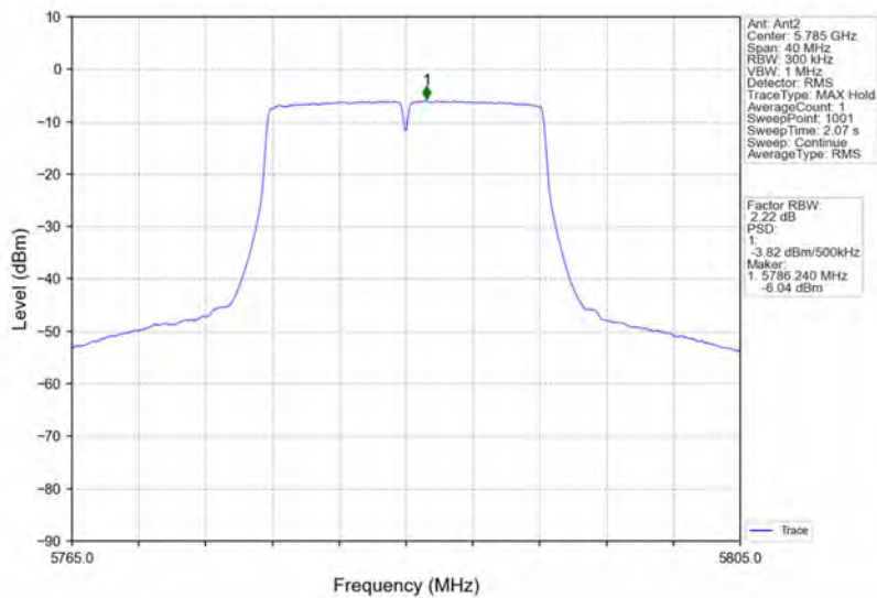
802.11a_MCH_5785MHz_Ant2_NTNV
