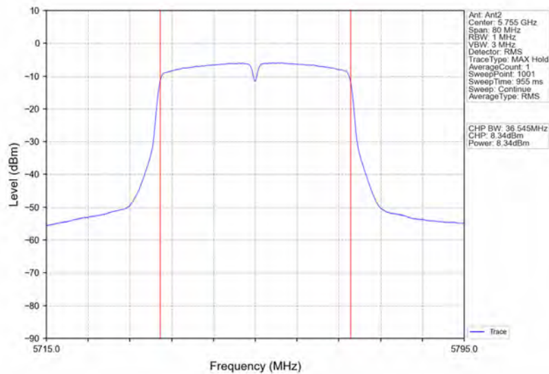
802.11ac(VHT40)_LCH_5755MHz_Ant2_NTNV
