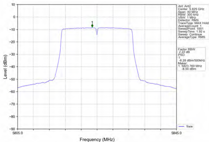
802.11n(HT20)_HCH_5825MHz_Ant2_NTNV
