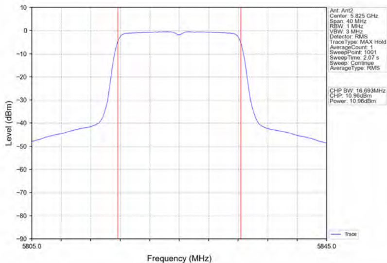
802.11a_HCH_5825MHz_Ant2_NTNV
