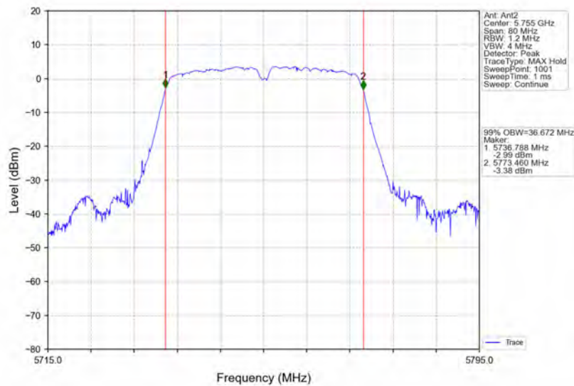
802.11n(HT40)_LCH_5755MHz_Ant2_NTNV
