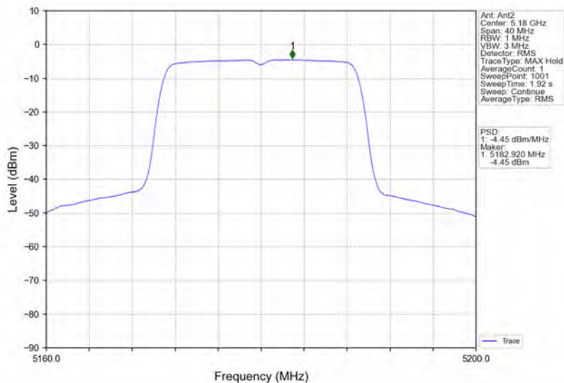
802.11n(HT20)_LCH_5180MHz_Ant2_NTNV
