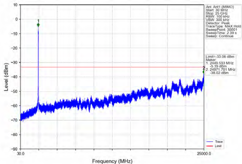
802.11n(HT40)_HCH_2452MHz_Ant1 (MIMO)_NTNV
