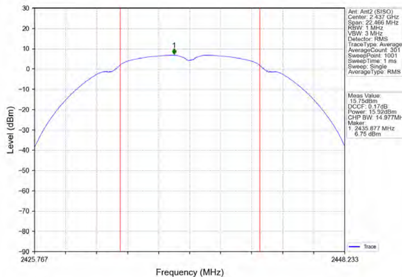
802.11b_MCH_2437MHz_Ant2 (SISO)_NTNV
