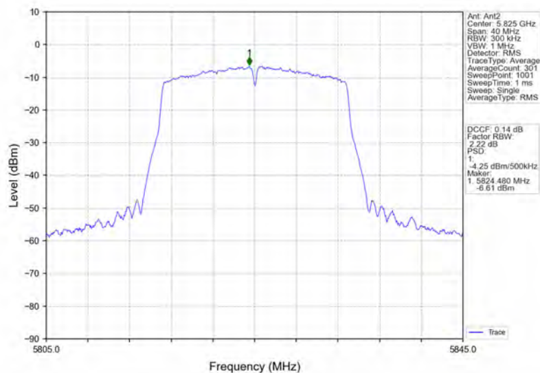
802.11n(HT20)_HCH_5825MHz_Ant2_NTNV
