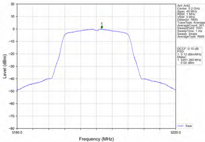
802.11a_MCH_5200MHz_Ant2_NTNV
