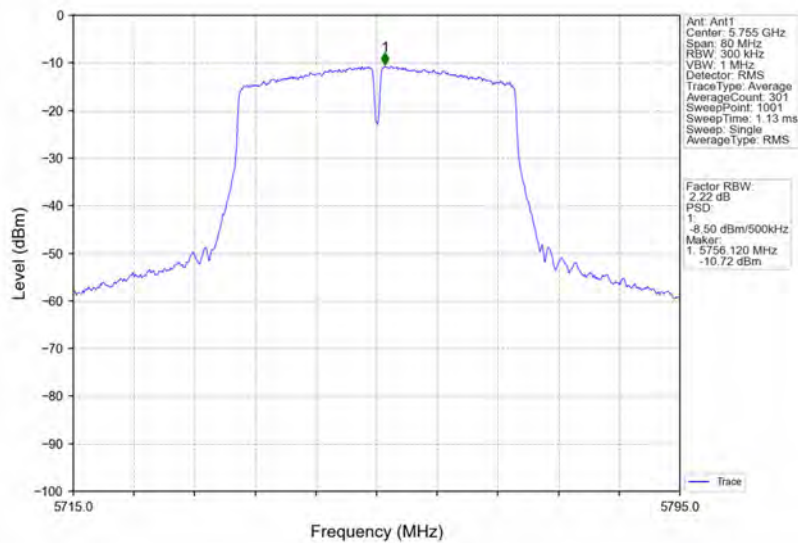
802.11n(HT40)_LCH_5755MHz_Ant1_NTNV
