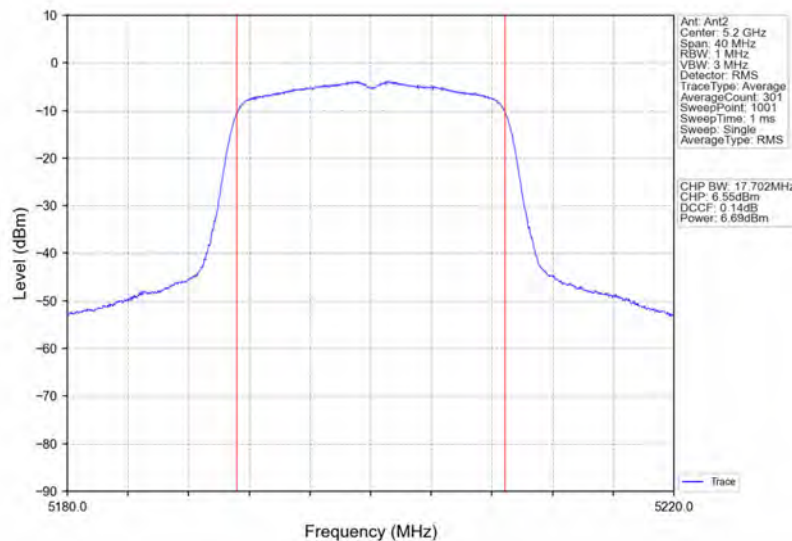
802.11n(HT20)_MCH_5200MHz_Ant2_NTNV
