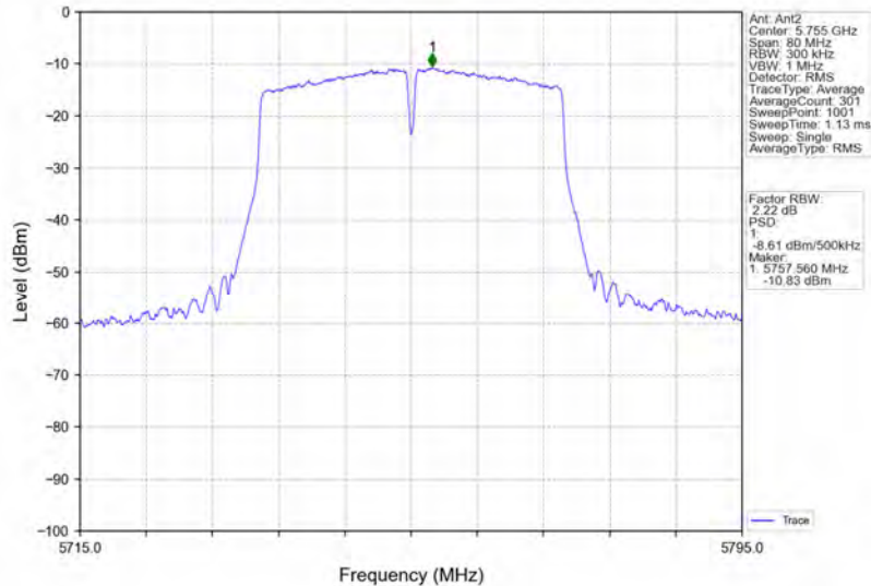
802.11n(HT40)_LCH_5755MHz_MIMO_NTNV
