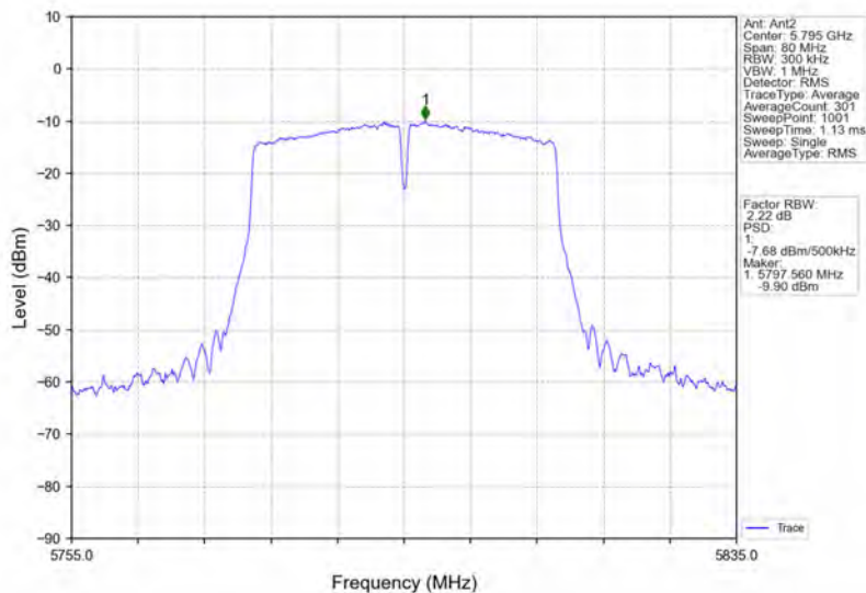
802.11n(HT40)_HCH_5795MHz_Ant2_NTNV
