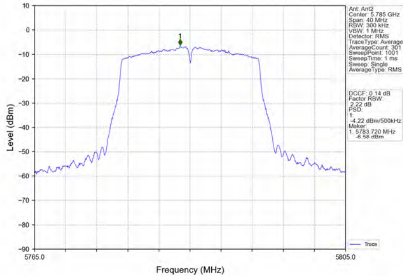
802.11n(HT20)_MCH_5785MHz_MIMO_NTNV
