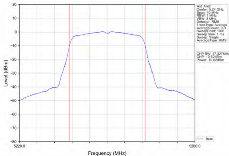
802.11a_HCH_5240MHz_Ant2_NTNV
