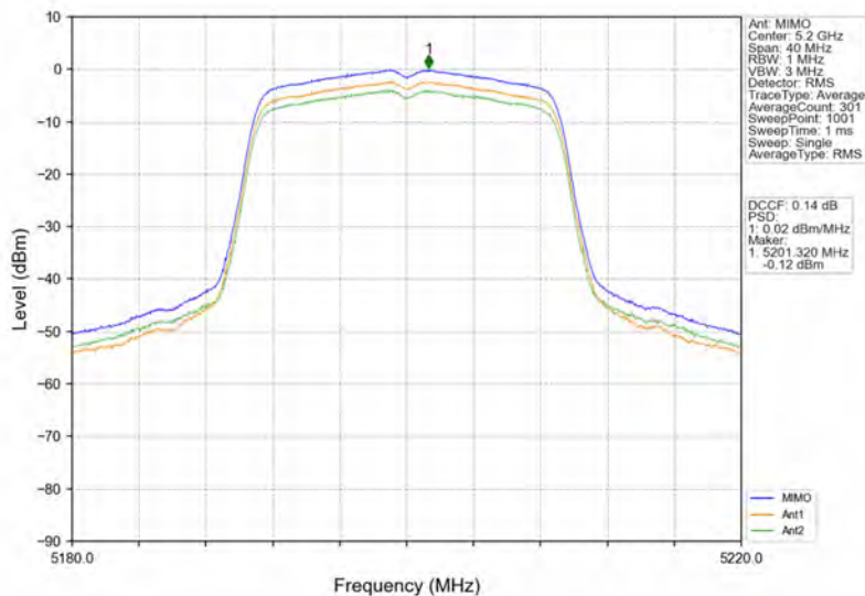
802.11n(HT20)_MCH_5200MHz_MIMO_NTNV
