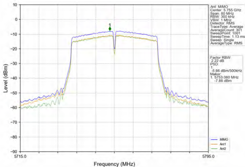
802.11n(HT40)_LCH_5755MHz_MIMO_NTNV
