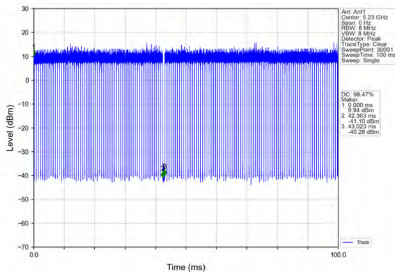
802.11n(HT40)_HCH_5230MHz_Ant1_NTNV
