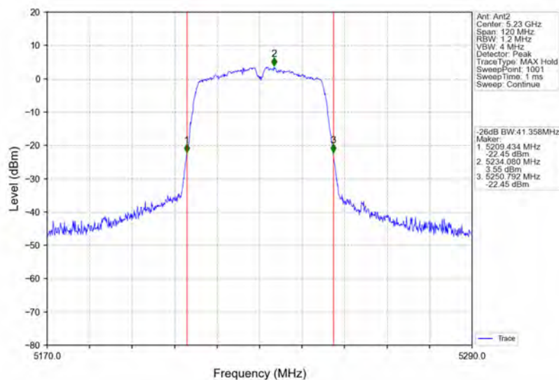
802.11n(HT40)_HCH_5230MHz_Ant2_NTNV
