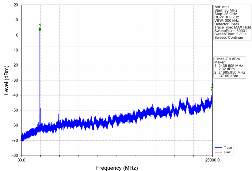
2M_MCH_2440MHz_Ant1_NTNV
