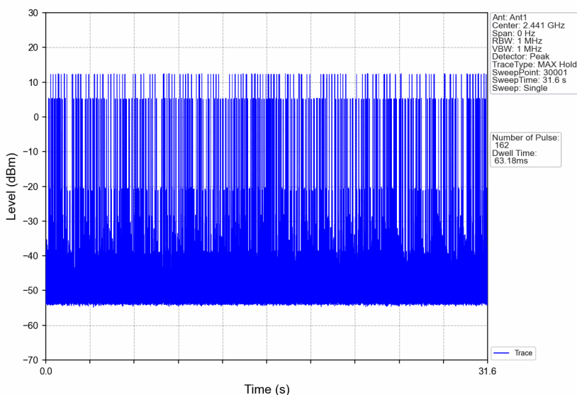
Pi/4DQPSK_2DH1_HOPP_Ant1_NTNV
