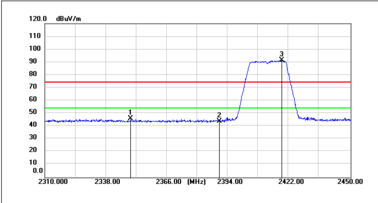
11n(HT20)_TX_CH_01_Horizontal_Peak
