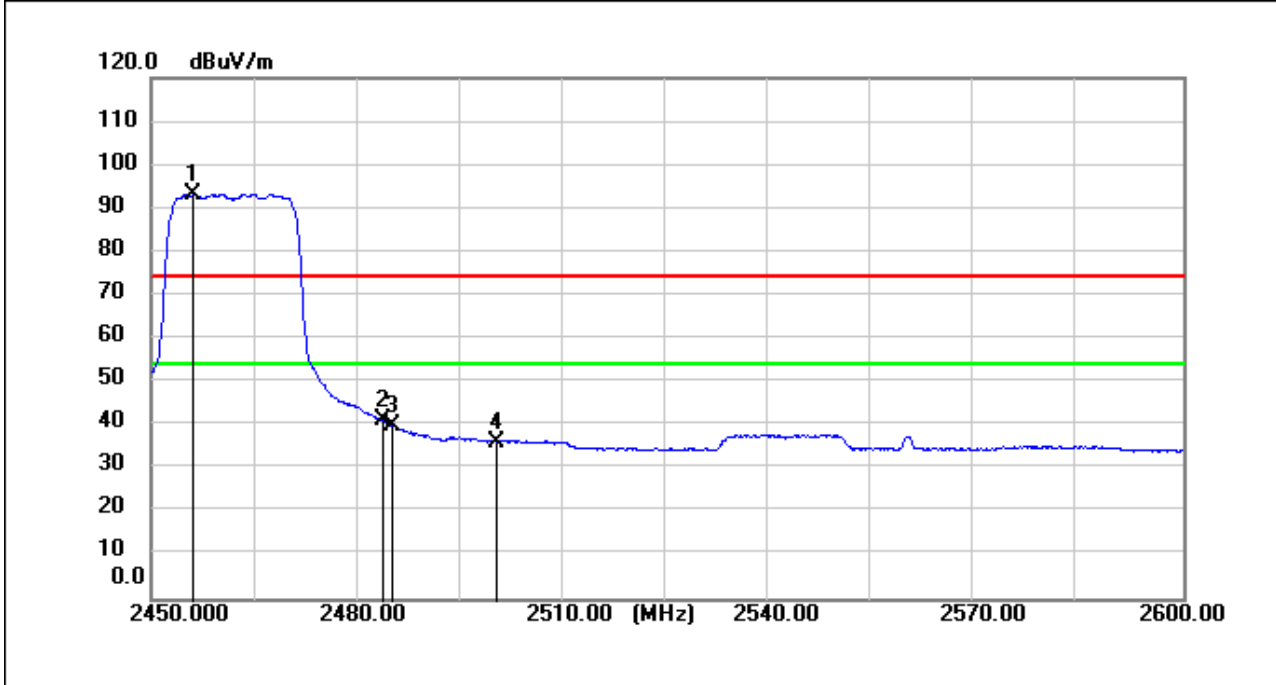
11n(HT20)_TX_CH_11_Vertical_Average
