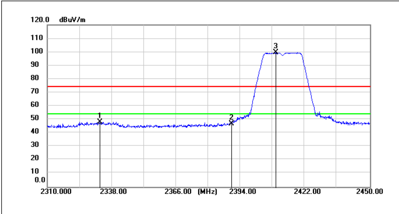
11n(HT20)_TX_CH_01_Vertical_Peak
