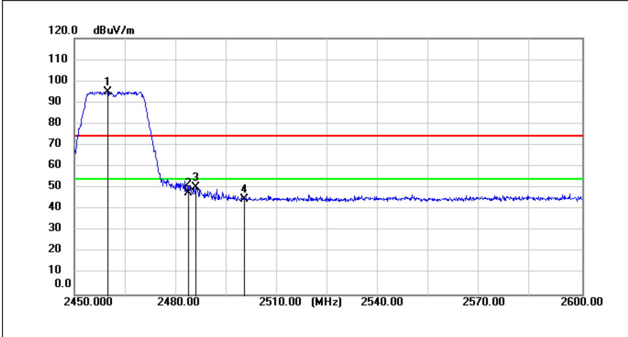
11n(HT20)_TX_CH_11_Horizontal_Peak
