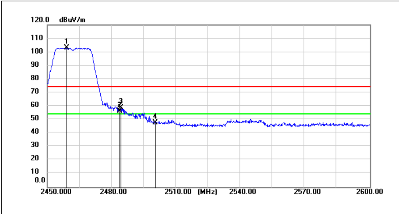
11n(HT20)_TX_CH_11_Vertical_Peak
