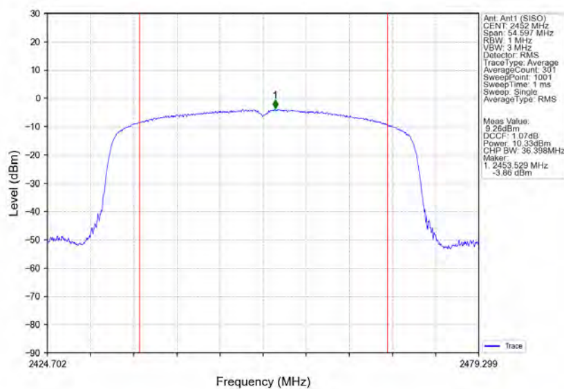
802.11ax(HEW40)_HCH_2452MHz_SU_/_Ant1 (SISO)_NTNV
