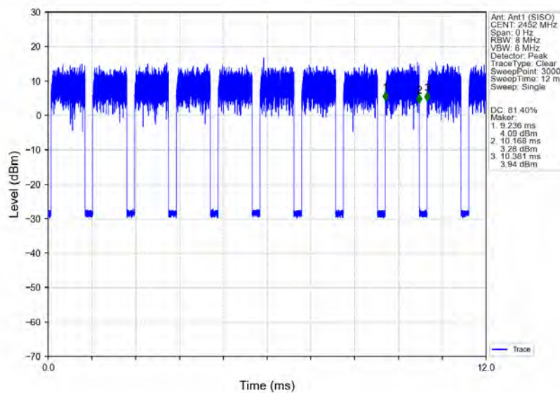
802.11n(HT40)_HCH_2452MHz_Ant1 (SISO)_NTNV
