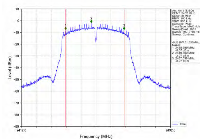
802.11n(HT40)_HCH_2452MHz_Ant1 (SISO)_NTNV
