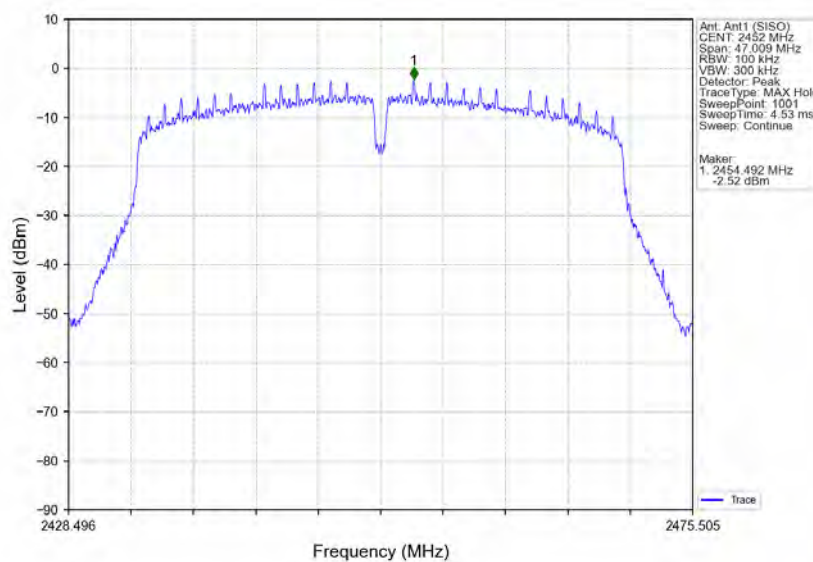
802.11n(HT40)_HCH_2452MHz_Ant1 (SISO)_NTNV
