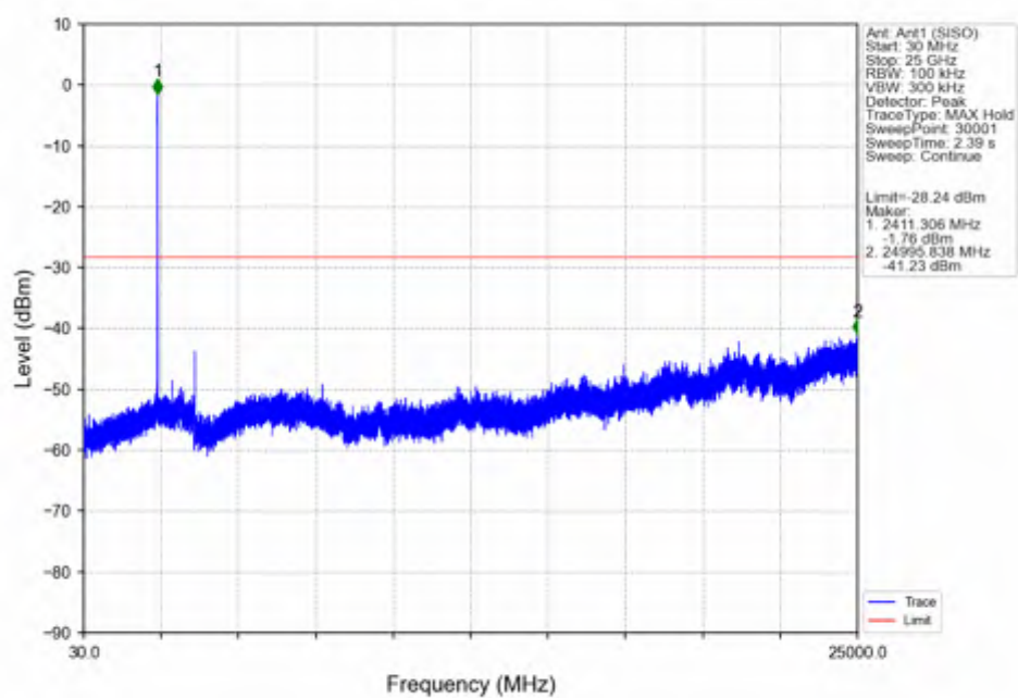
802.11n(HT20)_LCH_2412MHz_Ant1 (SISO)_NTNV
