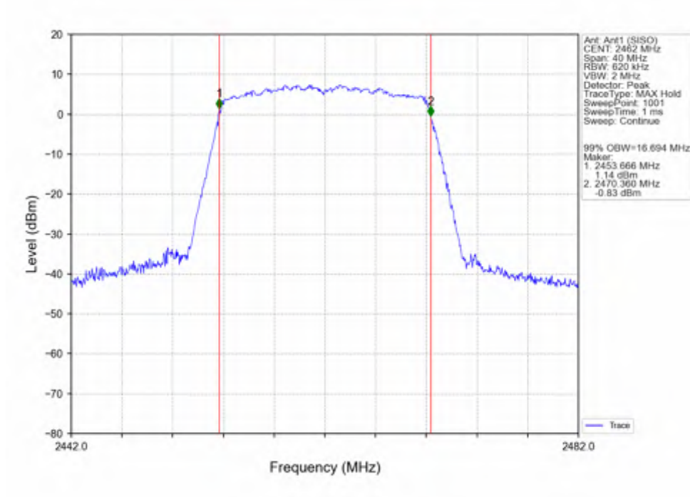
802.11g_HCH_2462MHz_Ant1 (SISO)_NTNV
