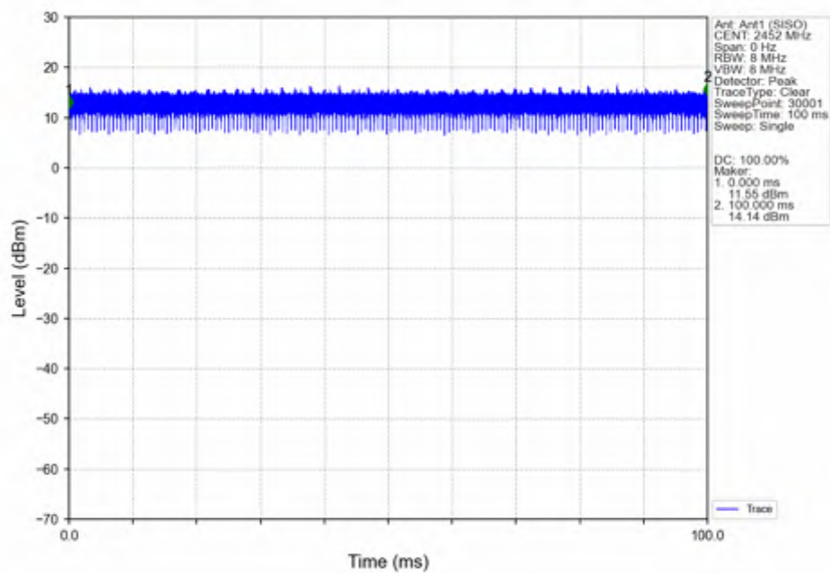
802.11n(HT40)_HCH_2452MHz_Ant1 (SISO)_NTNV
