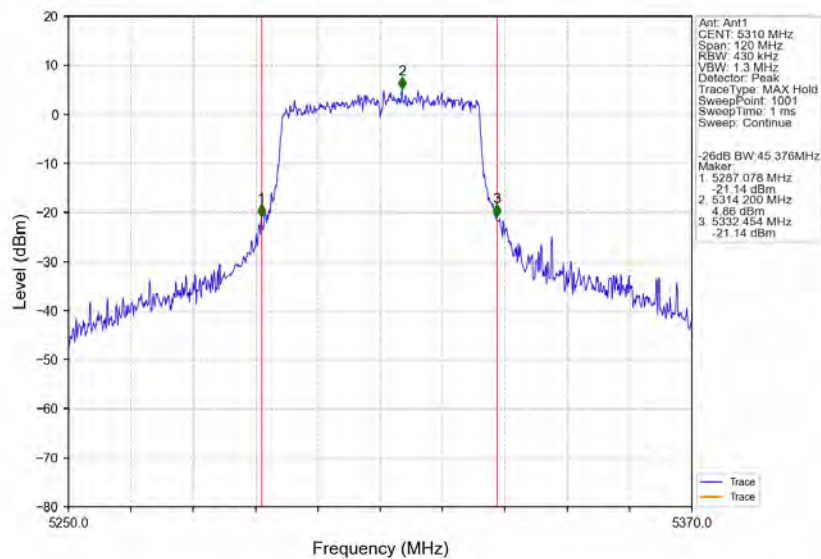
802.11ax(HE40) HCH 5310MHz RU484 Left Ant1 NTNv
