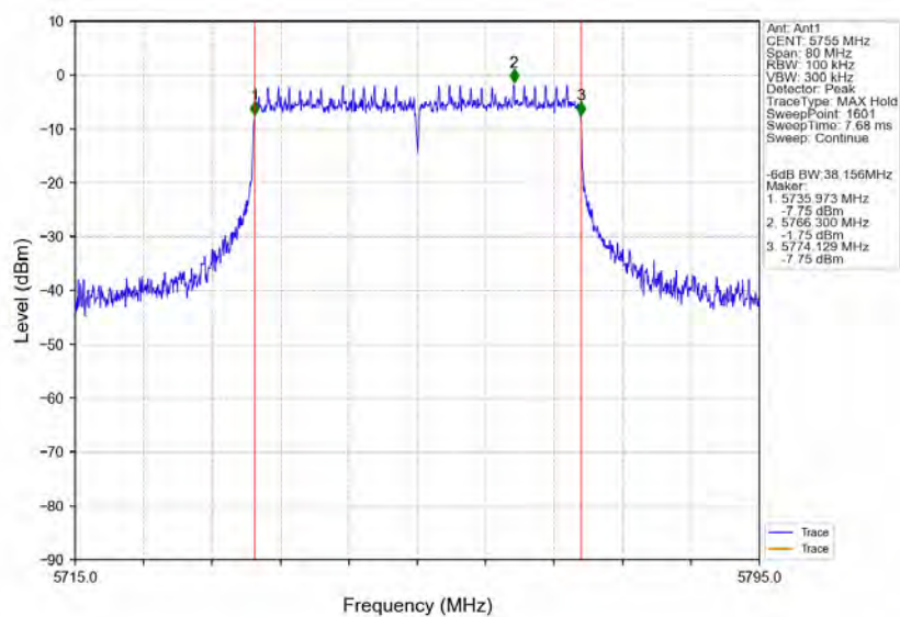
802.11ax(HE40) LCH 5755MHz RU484 Left Ant1 NTN
