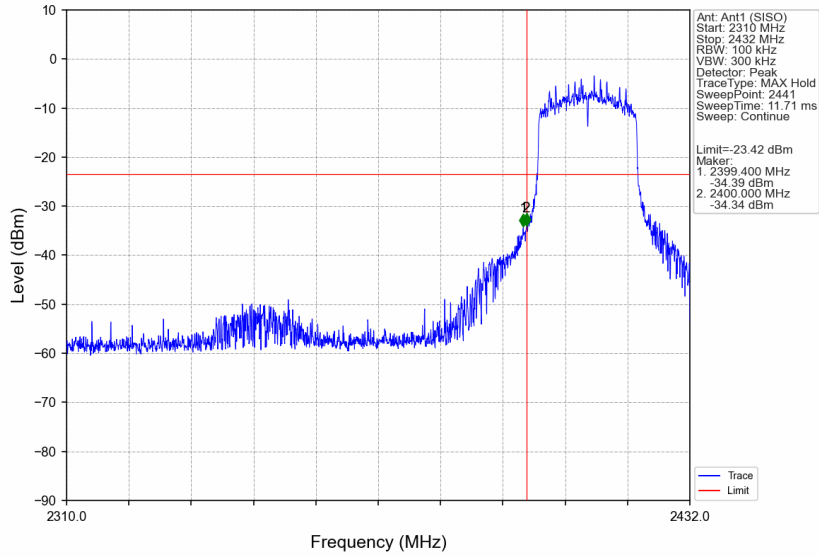
802.11ax(HE20)_LCH_2412MHz_RU242_Left_Ant1 (SISO)_NTNV
