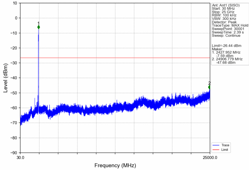
802.11ax(HE40)_MCH_2437MHz_RU484_Left_Ant1 (SISO)_NTNV
