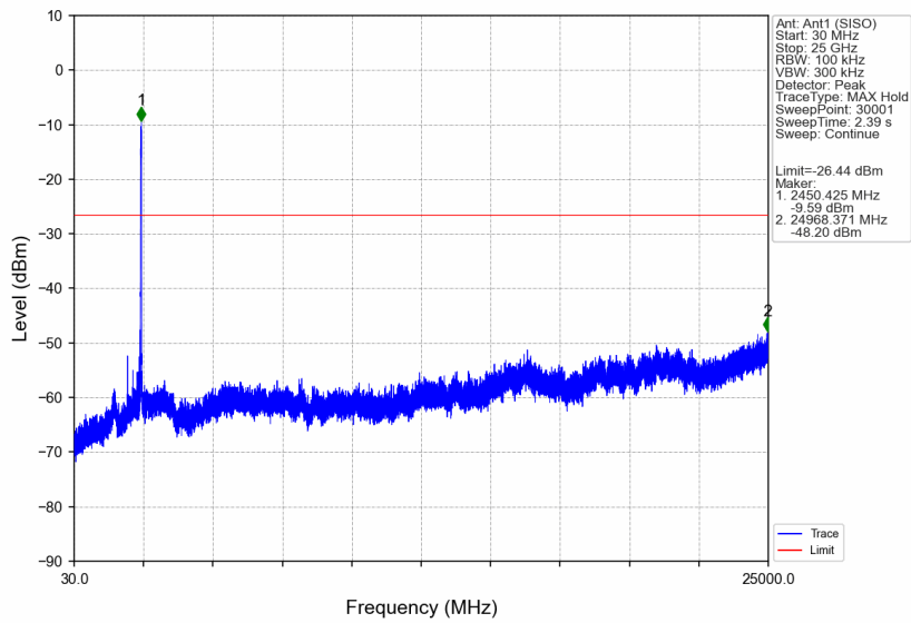
802.11ax(HE40)_MCH_2437MHz_RU484_Left_Ant1 (SISO)_NTNV
