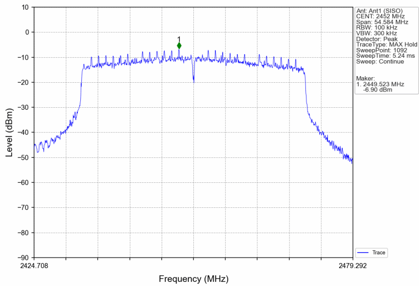
802.11ax(HE40)_HCH_2452MHz_RU484_Left_Ant1 (SISO)_NTNV
