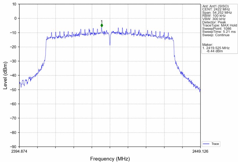
802.11ax(HE40)_LCH_2422MHz_RU484_Left_Ant1 (SISO)_NTNV
