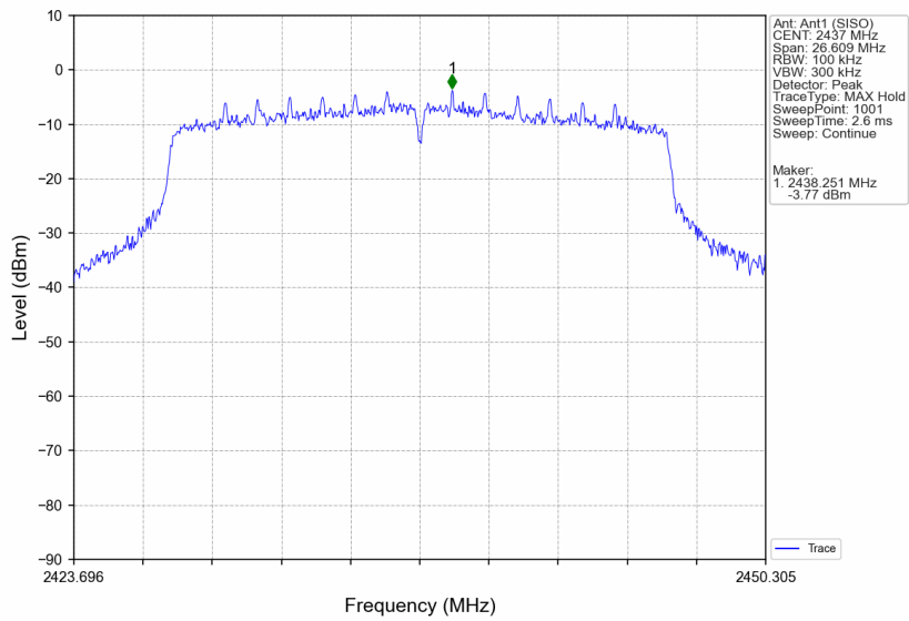
802.11ax(HE20)_MCH_2437MHz_RU242_Left_Ant1 (SISO)_NTNV
