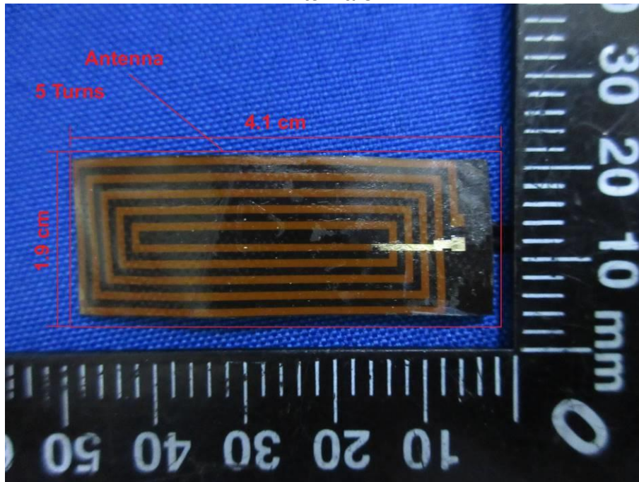
Antenna-3
