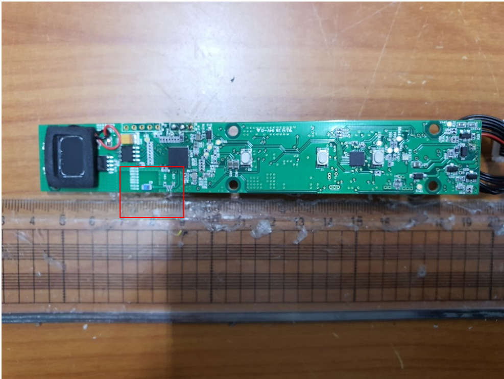
ANTENNA(2.4 GHz)
