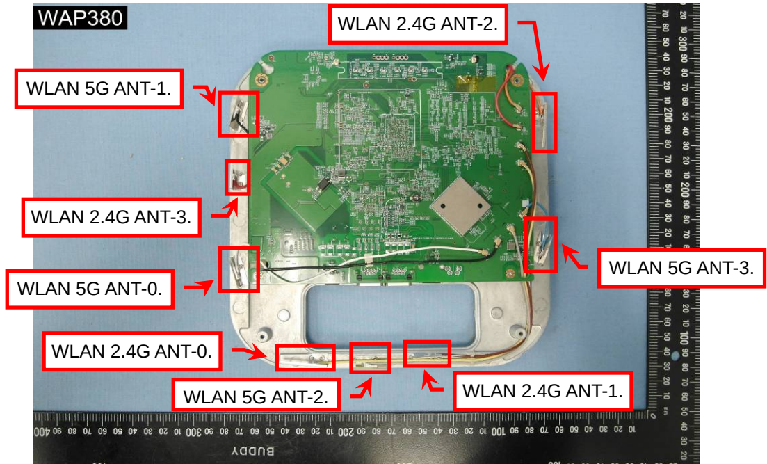
EUT Photo (12)
