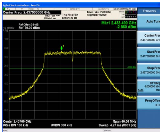
802.11n(HT20) CH06
