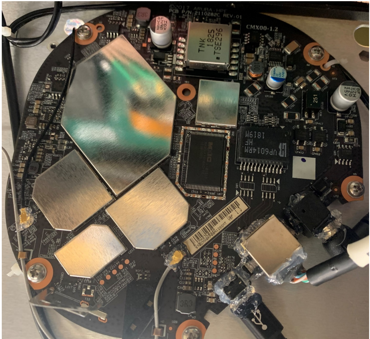
E14-625 Aruba Access Point (top)
