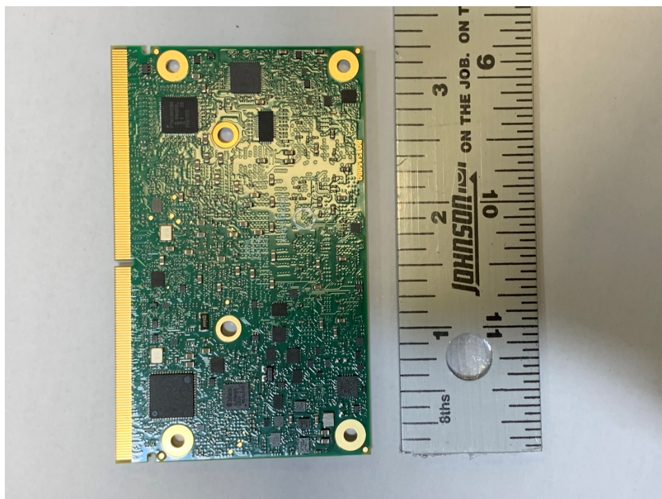
E14-631 Congatec (Back)
