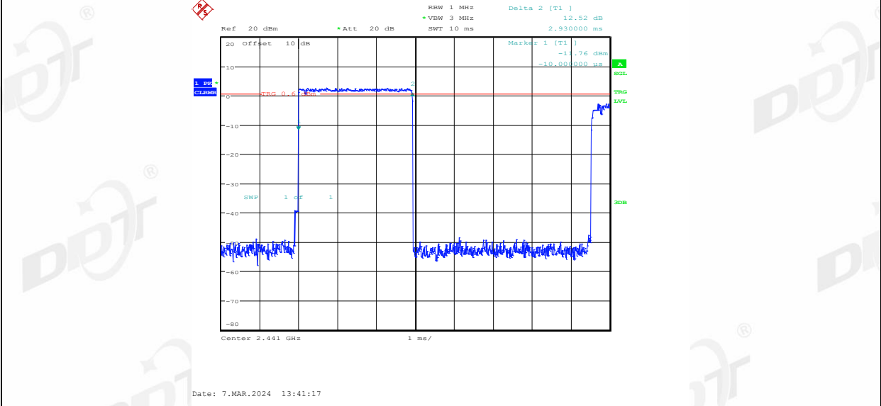
2DH5_Ant2_Hop
