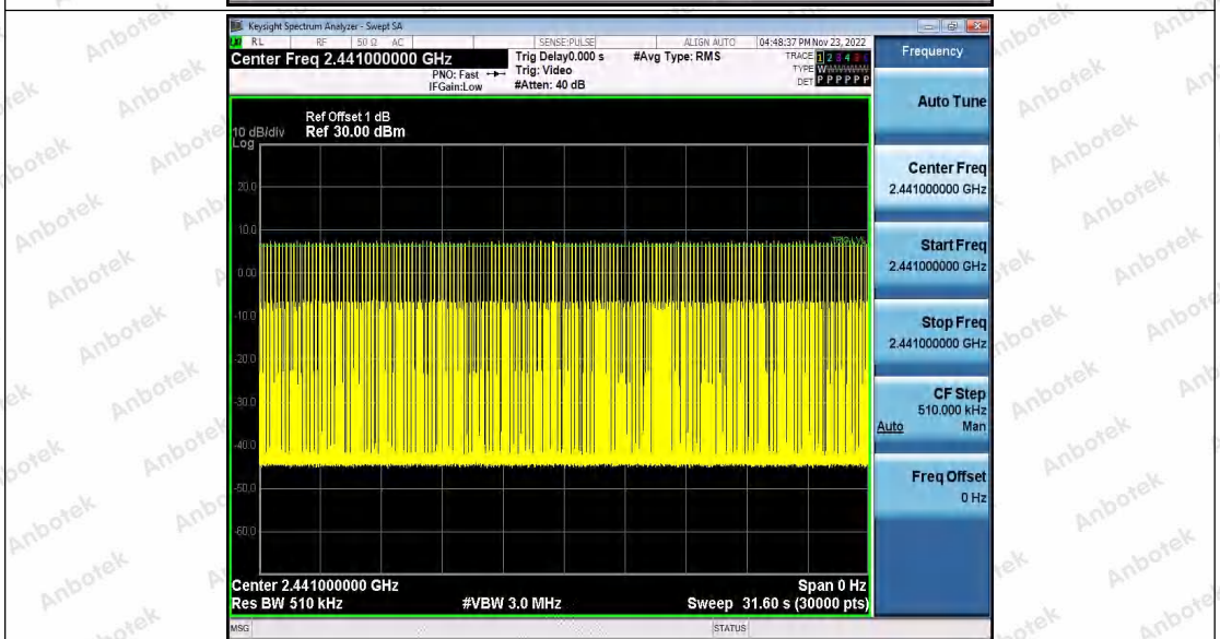
2DH3_Ant1_Hop
