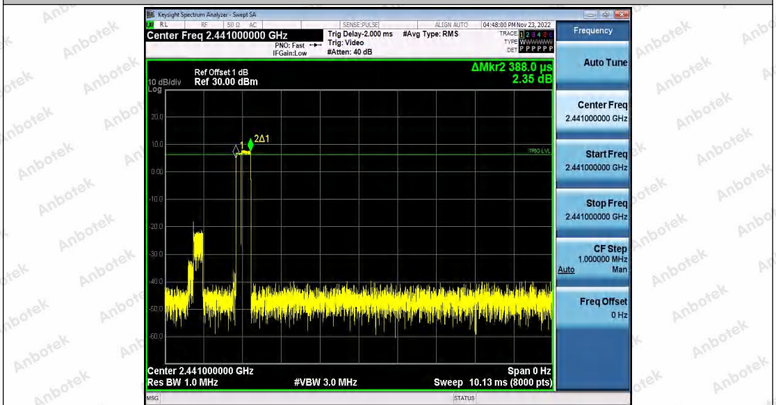
2DH1_Ant1_Hop
