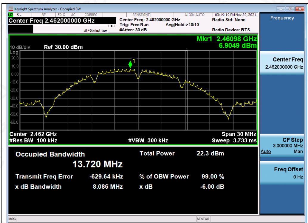
Test_Graph_802.11b_ANT1_2462_1Mbps_DTSBW
