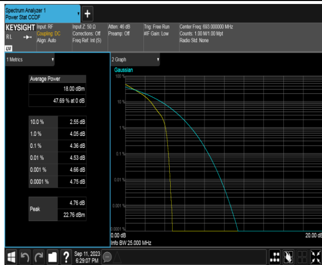
Band71-10MHz-QPSK-133422-50RB#0
