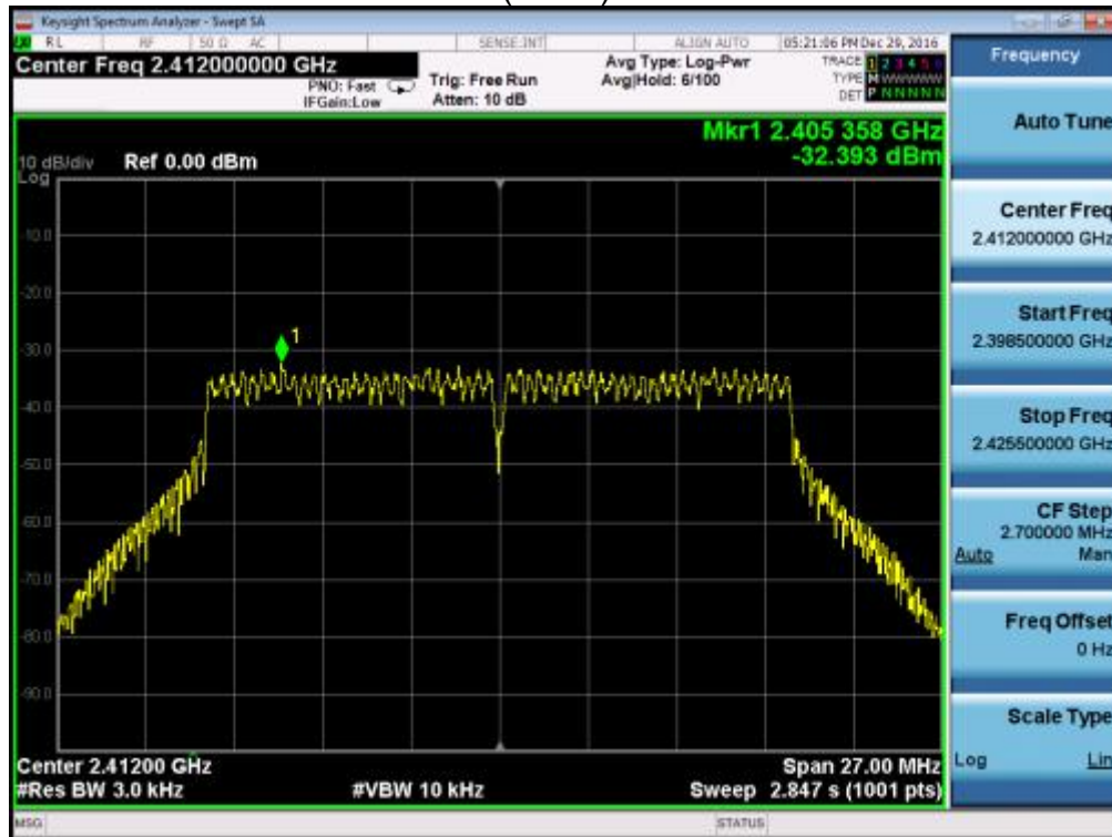
802.11n (HT20) 2412MHz
