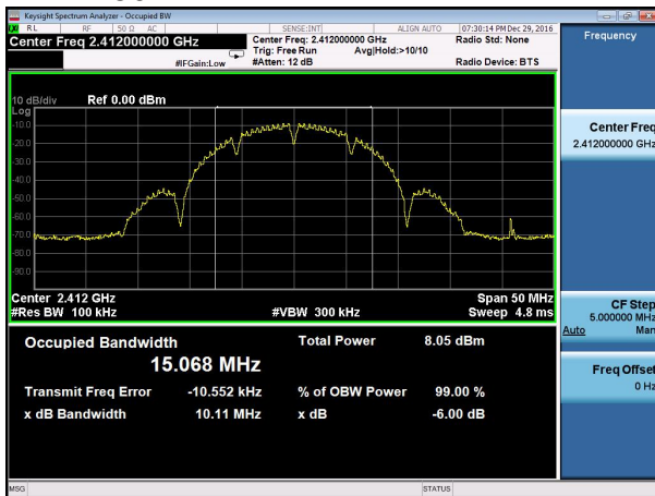
802.11b 2412MHz
