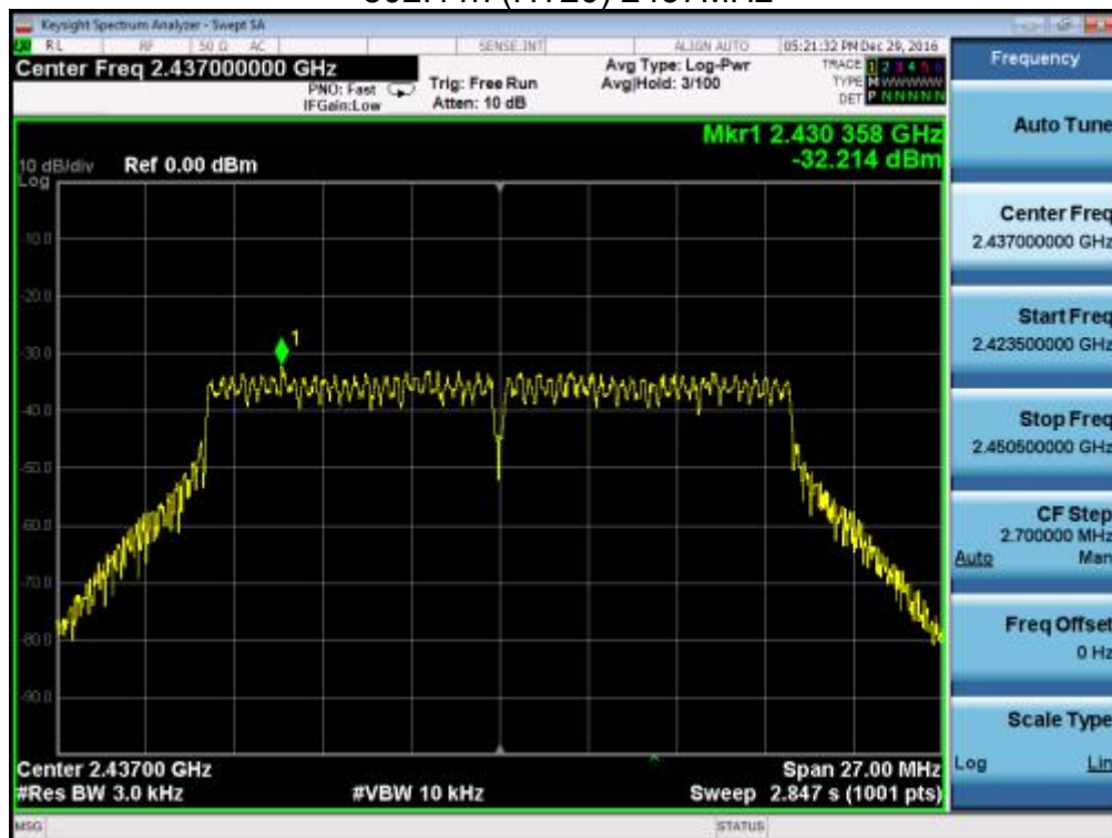
802.11n (HT20) 2437MHz
