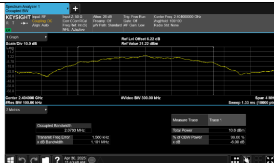
BLE 2M_Channel 1
