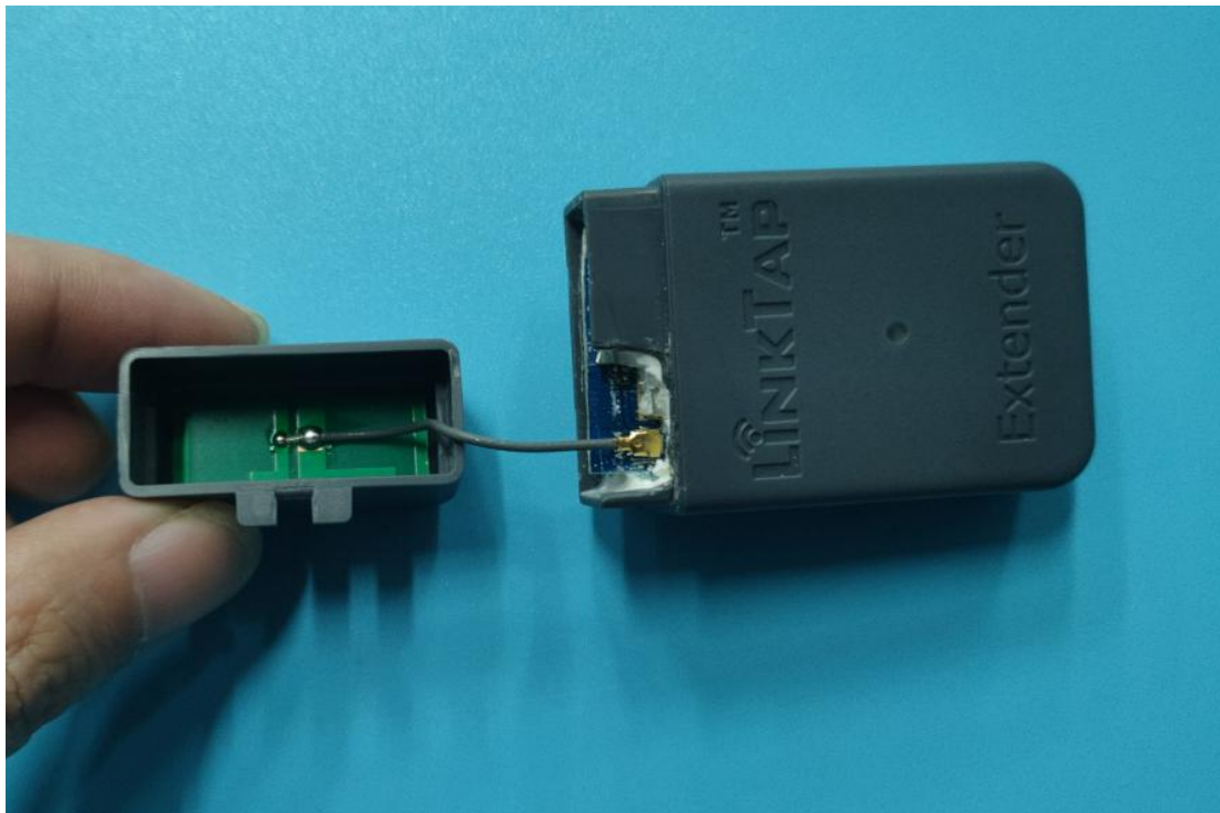
天线装配图
