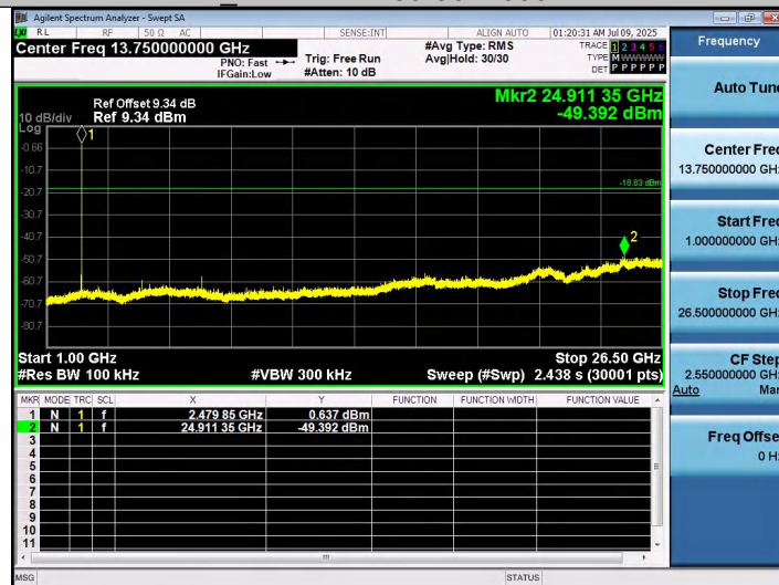
BLE 2M-Ant1-2480-1000~26500-PASS
