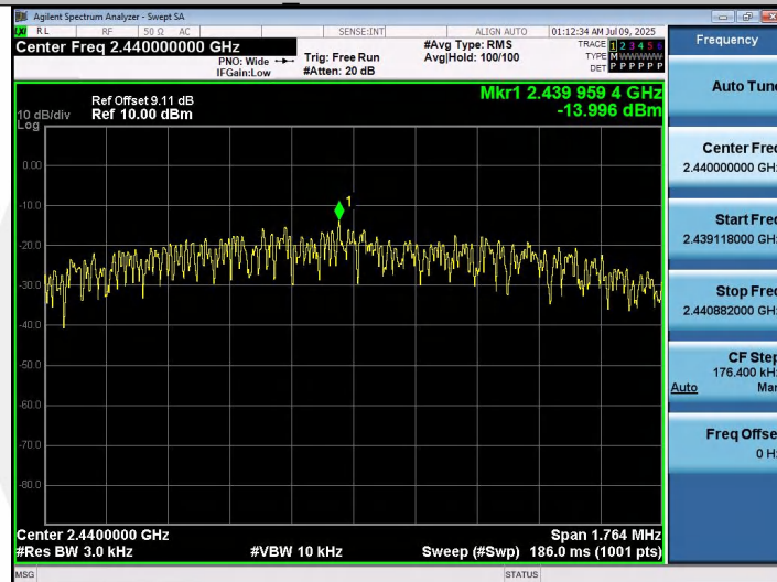
BLE 2M-Ant1-2440-PASS
