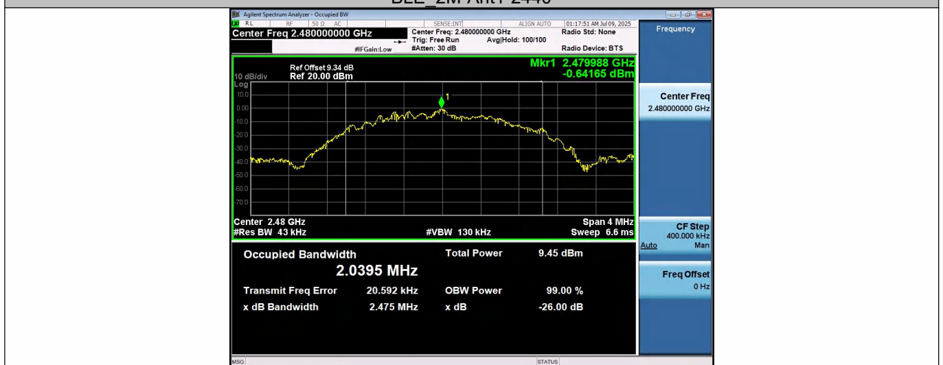
BLE 2M-Ant1-2480
