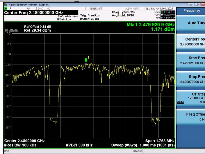
BLE 2M-Ant1-2480-PASS
