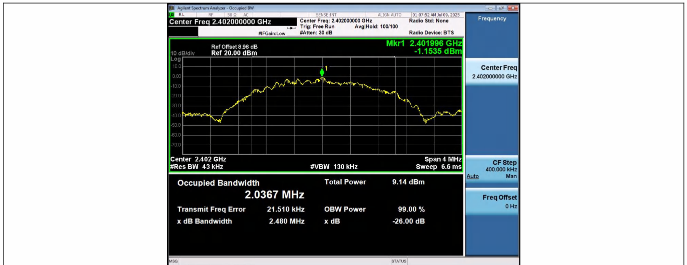
BLE 2M-Ant1-2402
