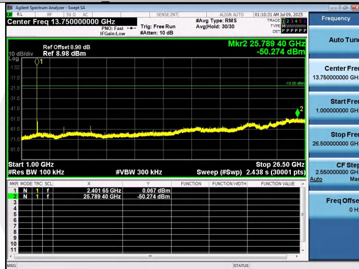
BLE 2M-Ant1-2402-1000~26500-PASS
