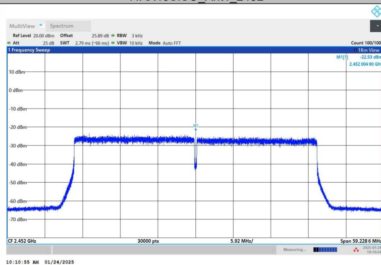
11AX40SISO_Ant1_2452
