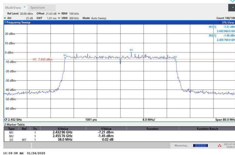
11AX40SISO_Ant1_2452
