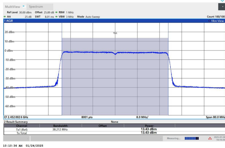
11AX40SISO_Ant1_2452
