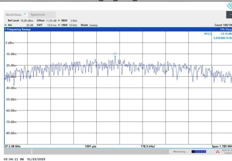
BLE_2M_Ant1_2480
