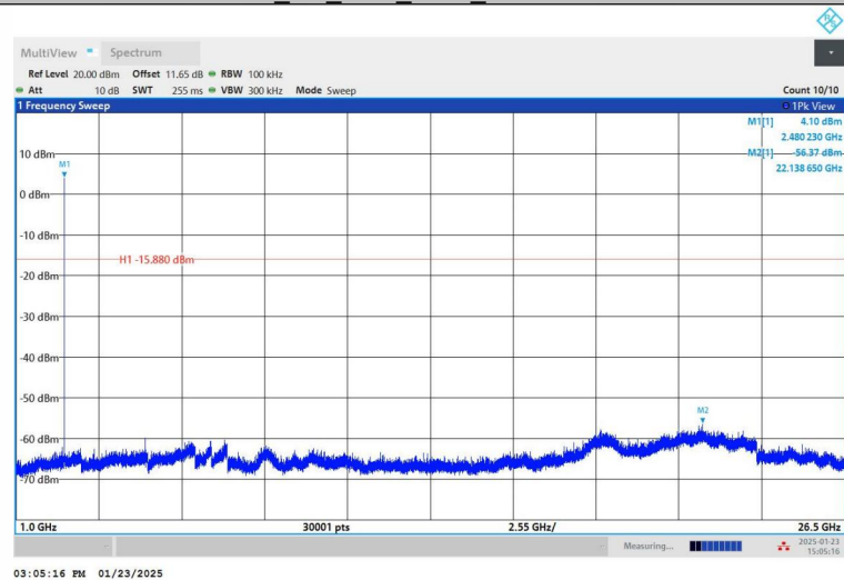
BLE_2M_Ant1_2480_1000~26500
