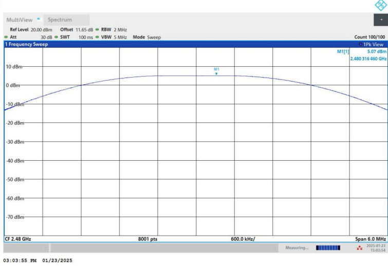
BLE_2M_Ant1_2480
