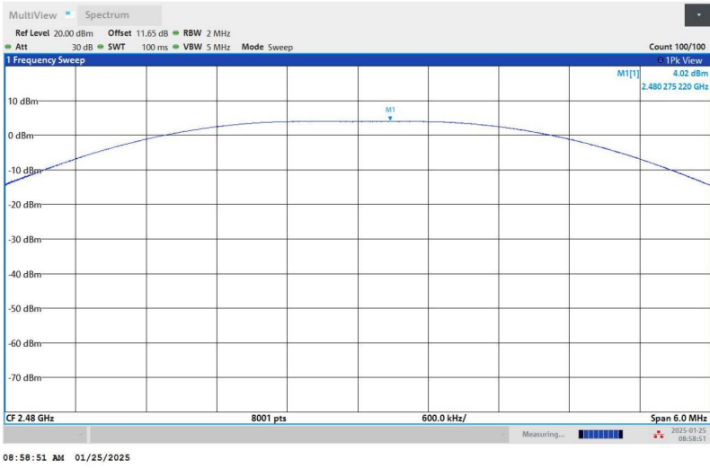
BLE_2M_Ant1_2480
