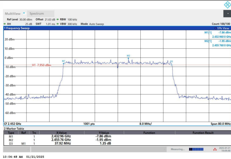
11AX40SISO_Ant1_2452
