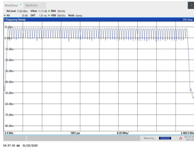
2DH5_Ant1_Hop
