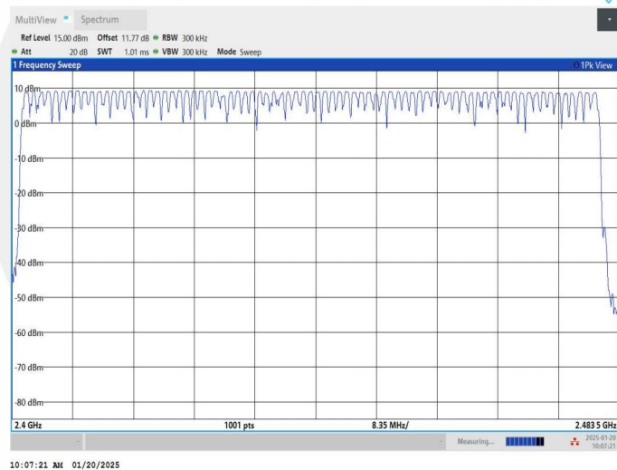
3DH5_Ant1_Hop
