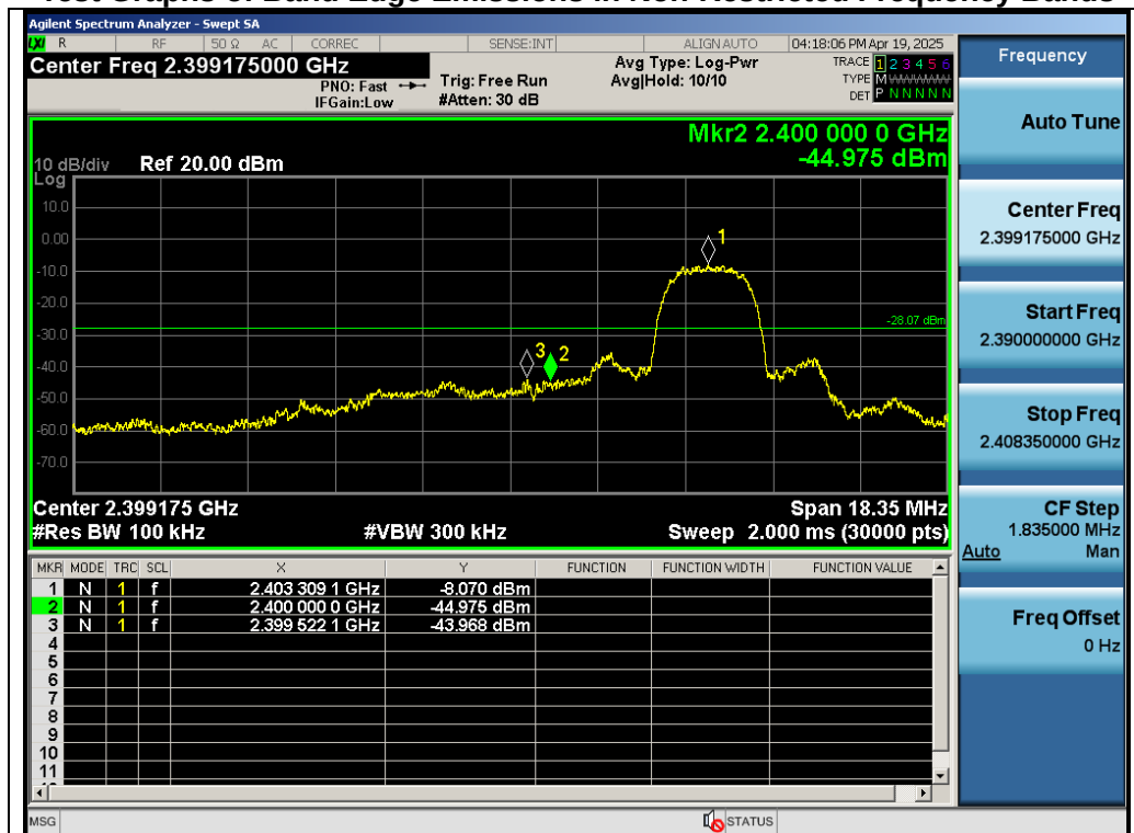
Test_Graph_SRD 2.4G_ANT0_2403.35_Lower Band Edge Emissions
