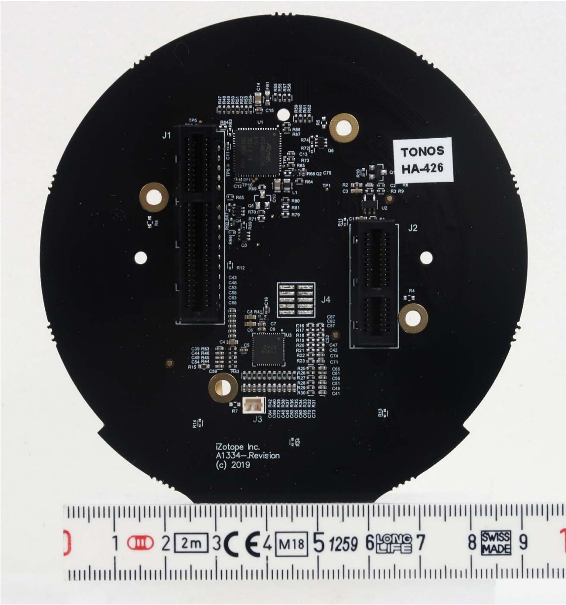
Tonos HA – 426 UI Module Side 2
