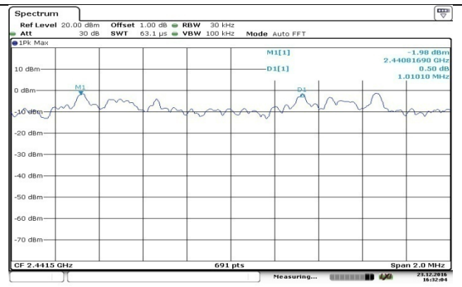
\pi/4 DQPSK
