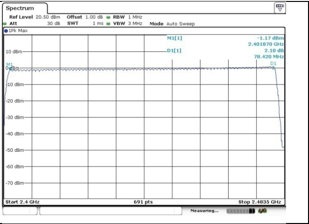
\pi/4 DQPSK
