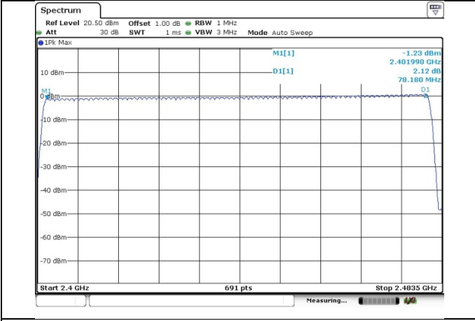
8DPSK
