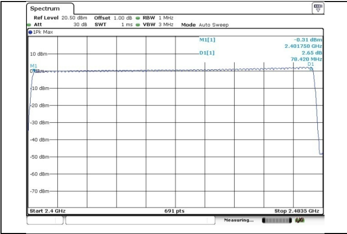
GFSK
