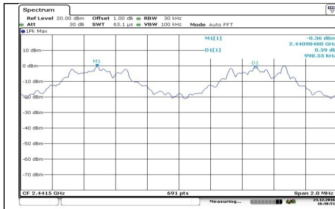
GFSK
