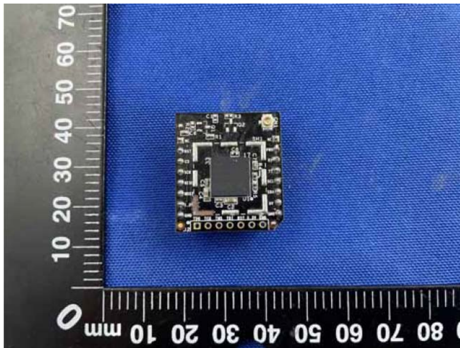
ZWAVE MODULE TOP VIEW ---2# circuit
