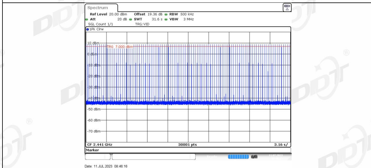
3DH1_Ant1_Hop
