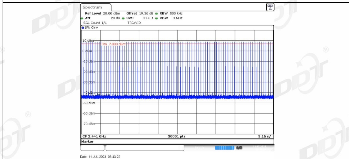
2DH1_Ant1_Hop
