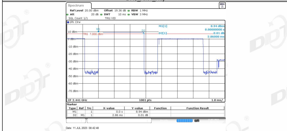
DH5_Ant1_Hop
