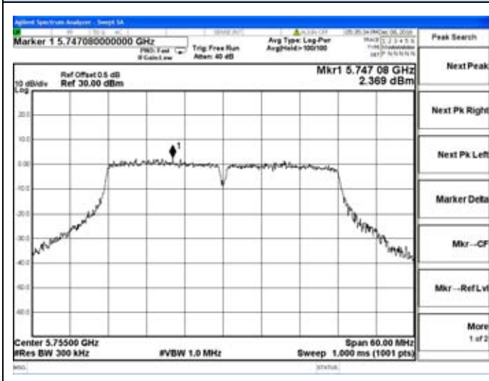
Chain 0-802.11n40-5755MHz
