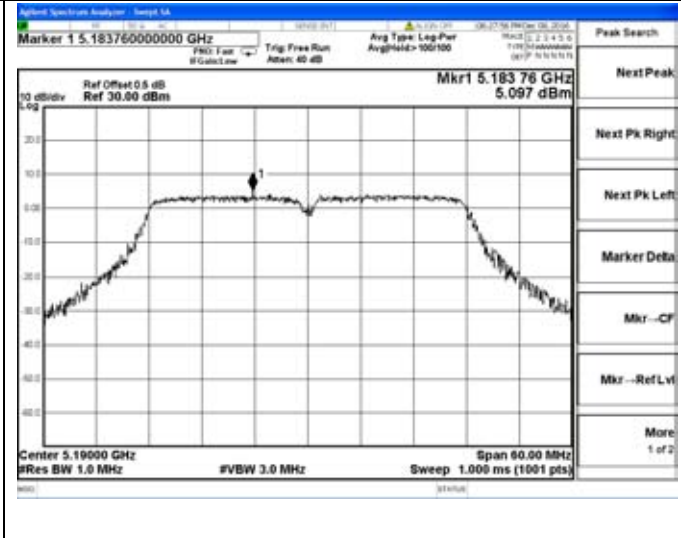
Chain 1-802.11n40-5190MHz
