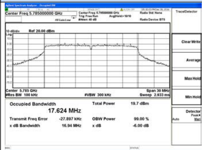
802.11n20-5785MHz
