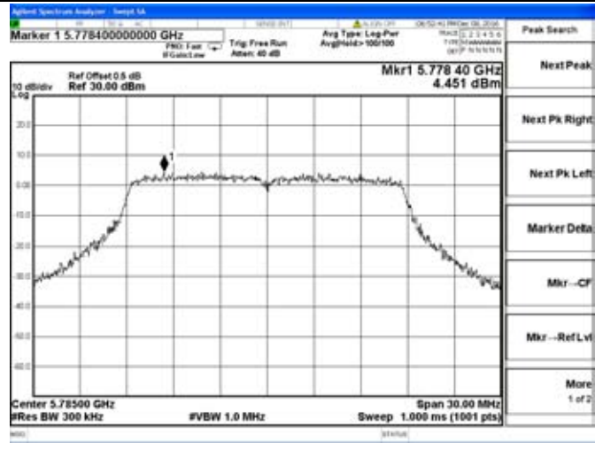
Chain 1-802.11n20-5785MHz
