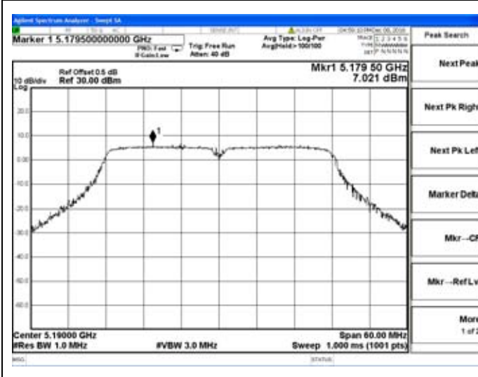
Chain 0-802.11n40-5190MHz
