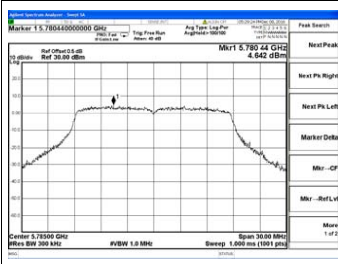
Chain 0-802.11n20-5785MHz
