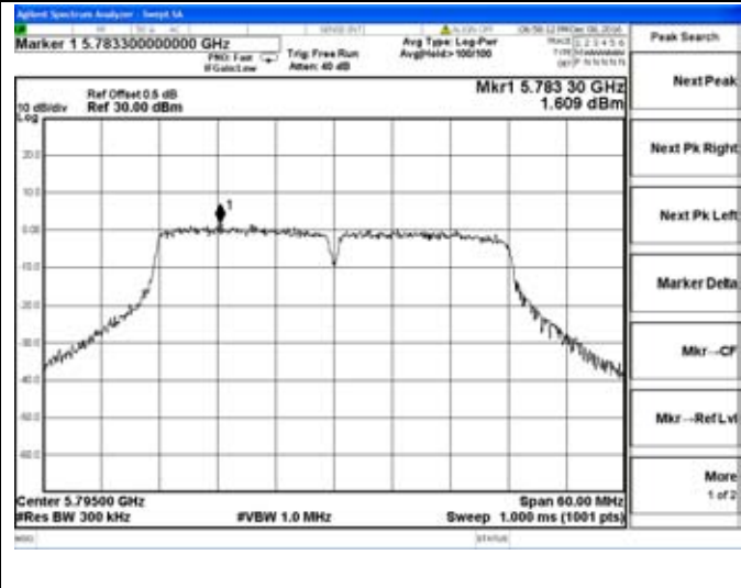
Chain 1-802.11n40-5795MHz
