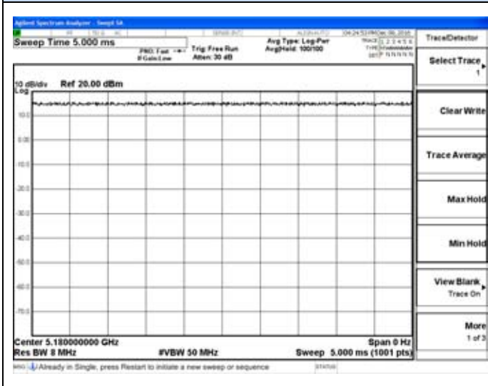
a-5180MHz
