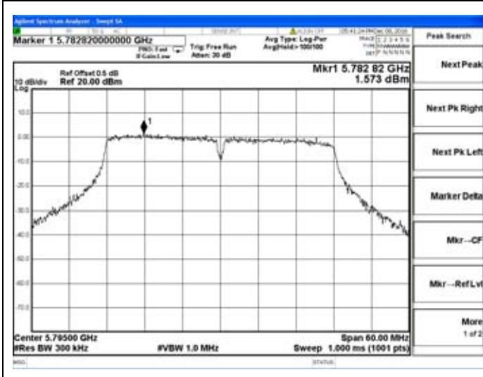
Chain 0-802.11n40-5795MHz
