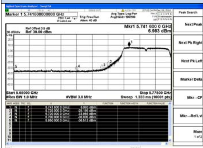
802.11n40-5755MHz-Lower
