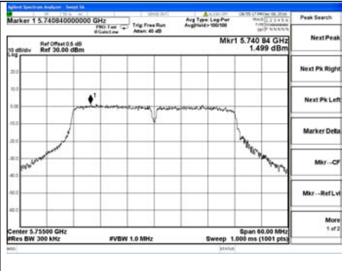
Chain 1-802.11n40-5755MHz
