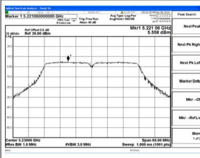
Chain 0-802.11n40-5230MHz
