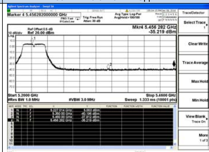
802.11n40-5230MHz-Upper
