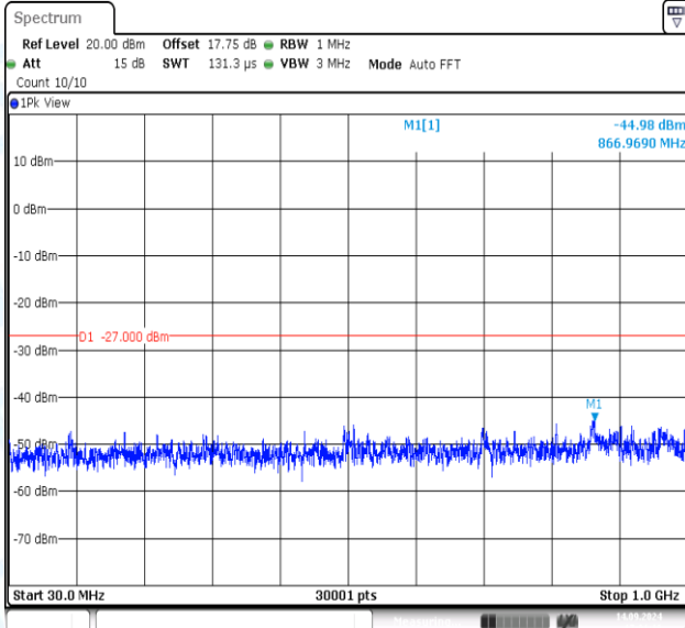
11N20MIMO-Ant1-5745-30~1000-PASS
