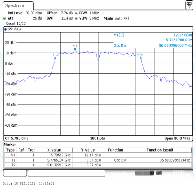
11N40MIMO-Ant2-5795
