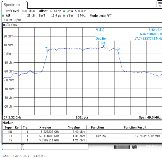
11N20MIMO-Ant1-5320
