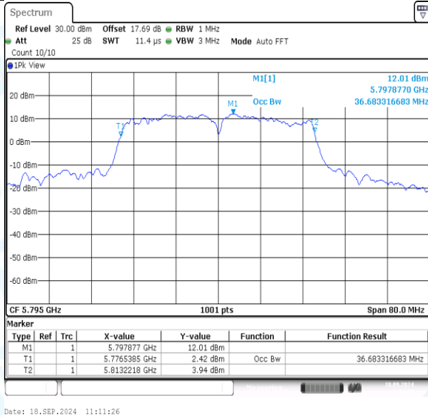
11N40MIMO-Ant1-5795
