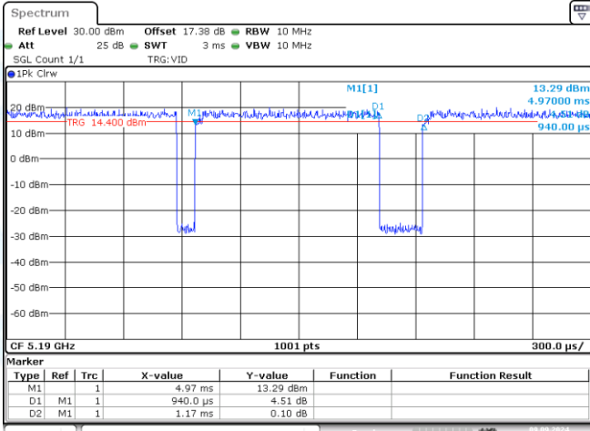
NTNV-11N40MIMO-Ant1-5190
