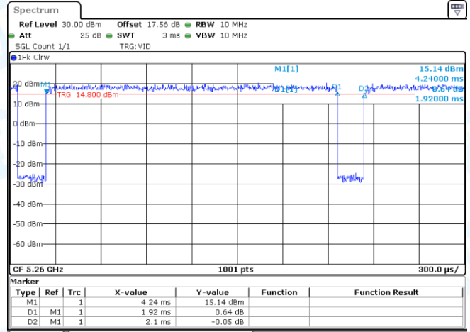
NTNV-11N20MIMO-Ant2-5260
