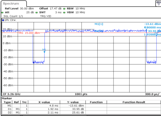
NTNV-11N20MIMO-Ant1-5260
