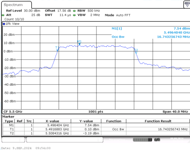
11A-Ant1-5500
