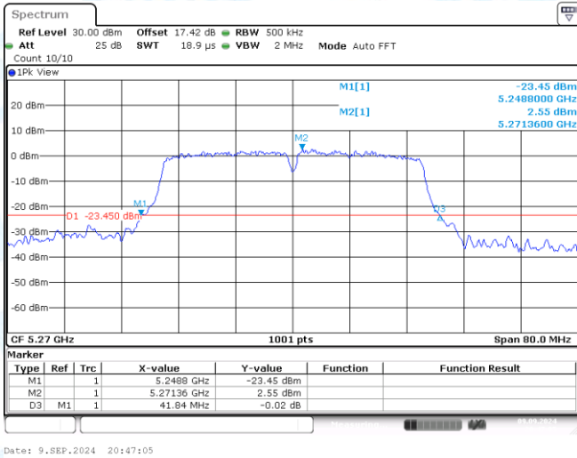
11AC40MIMO-Ant1-5270
