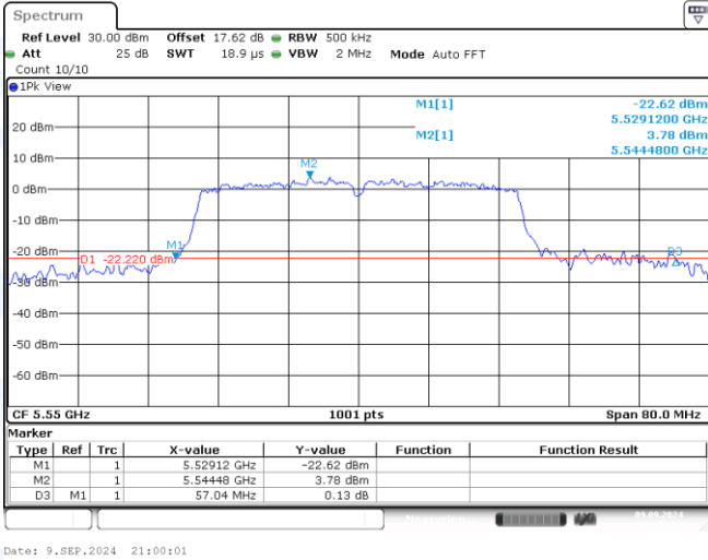
11AC40MIMO-Ant1-5550
