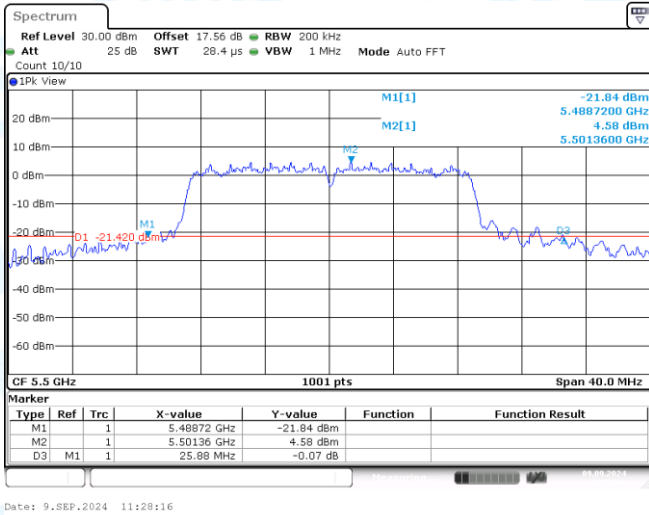
11N20MIMO-Ant1-5500
