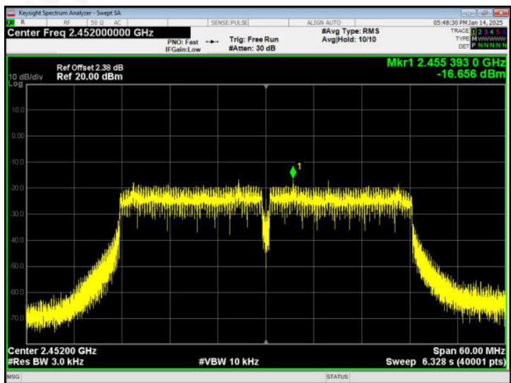
802.11n40 - CH09
