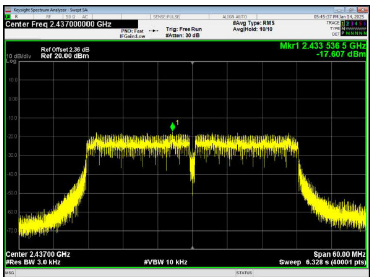
802.11n40 - CH06
