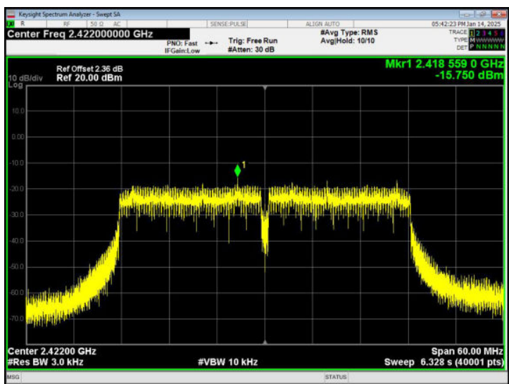
802.11n40 - CH03
