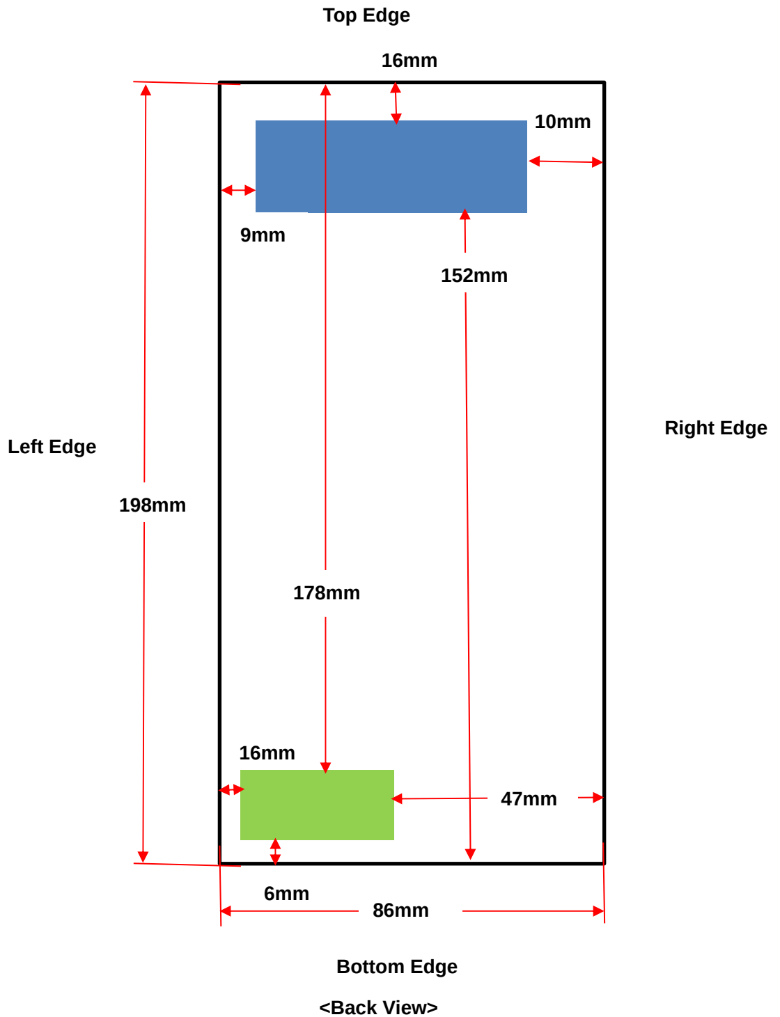
WWAN Antenna
