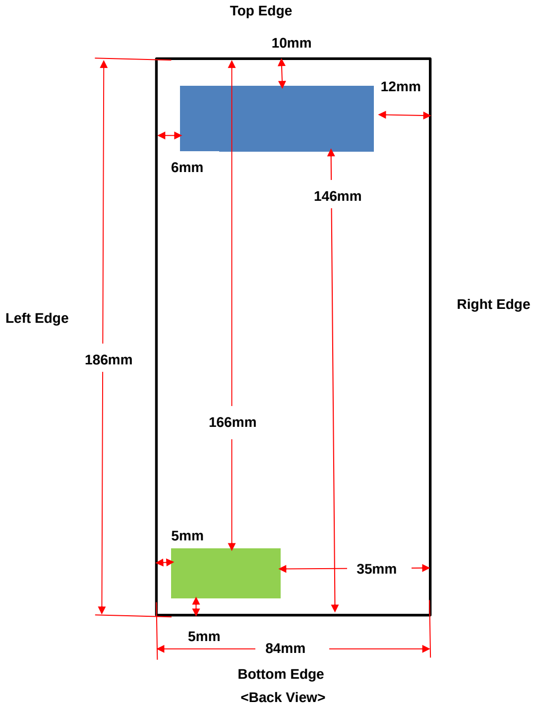
WWAN Antenna
