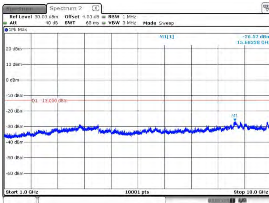
B26_CH26740_1.4M_1RB2_QPSK_Above 1G
