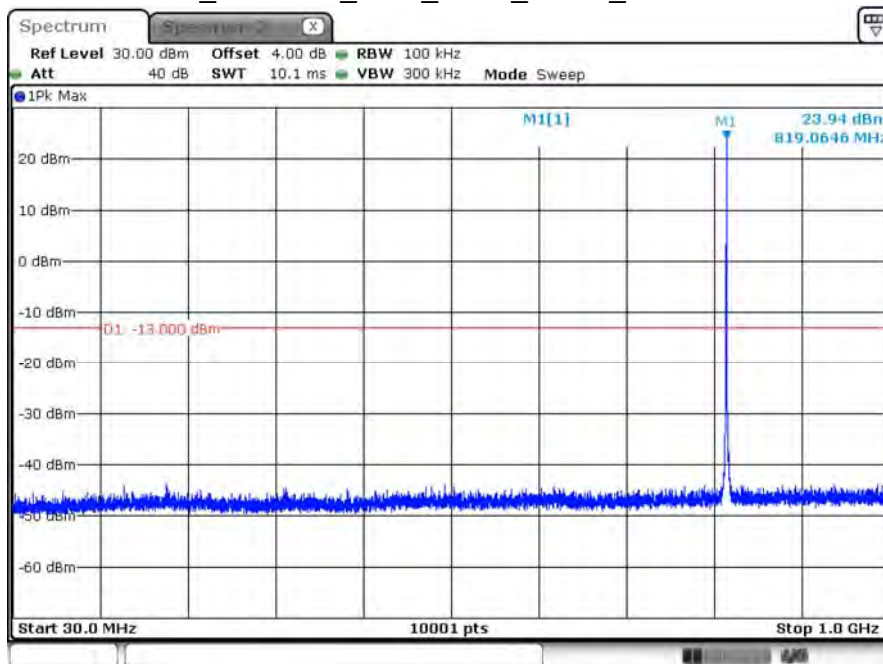
B26_CH26740_1.4M_1RB2_QPSK_Below 1G
