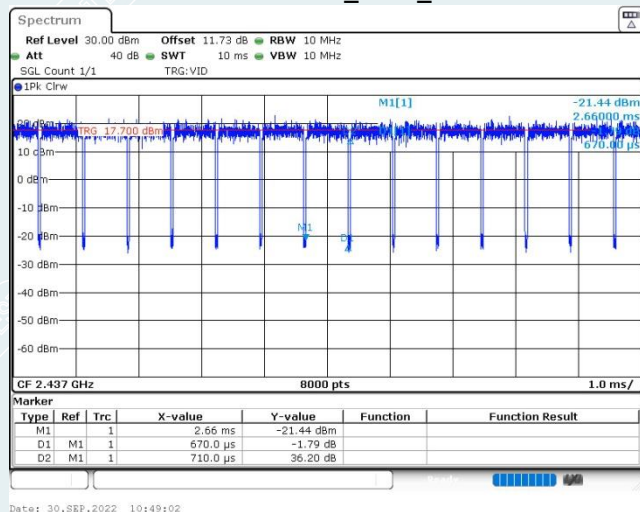
IEEE 802.11n HT20_Ant1_2437MHz
