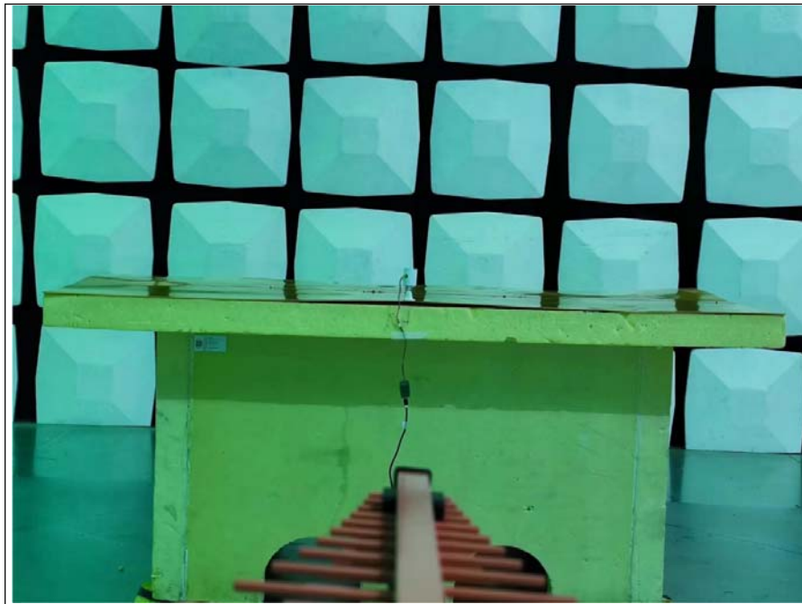
30MHz-1GHz(FCC&IC)
