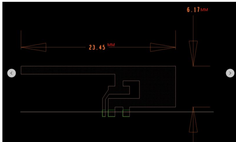
BLE antenna
